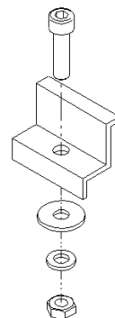
Figura 2: Morsetti di fissaggio
