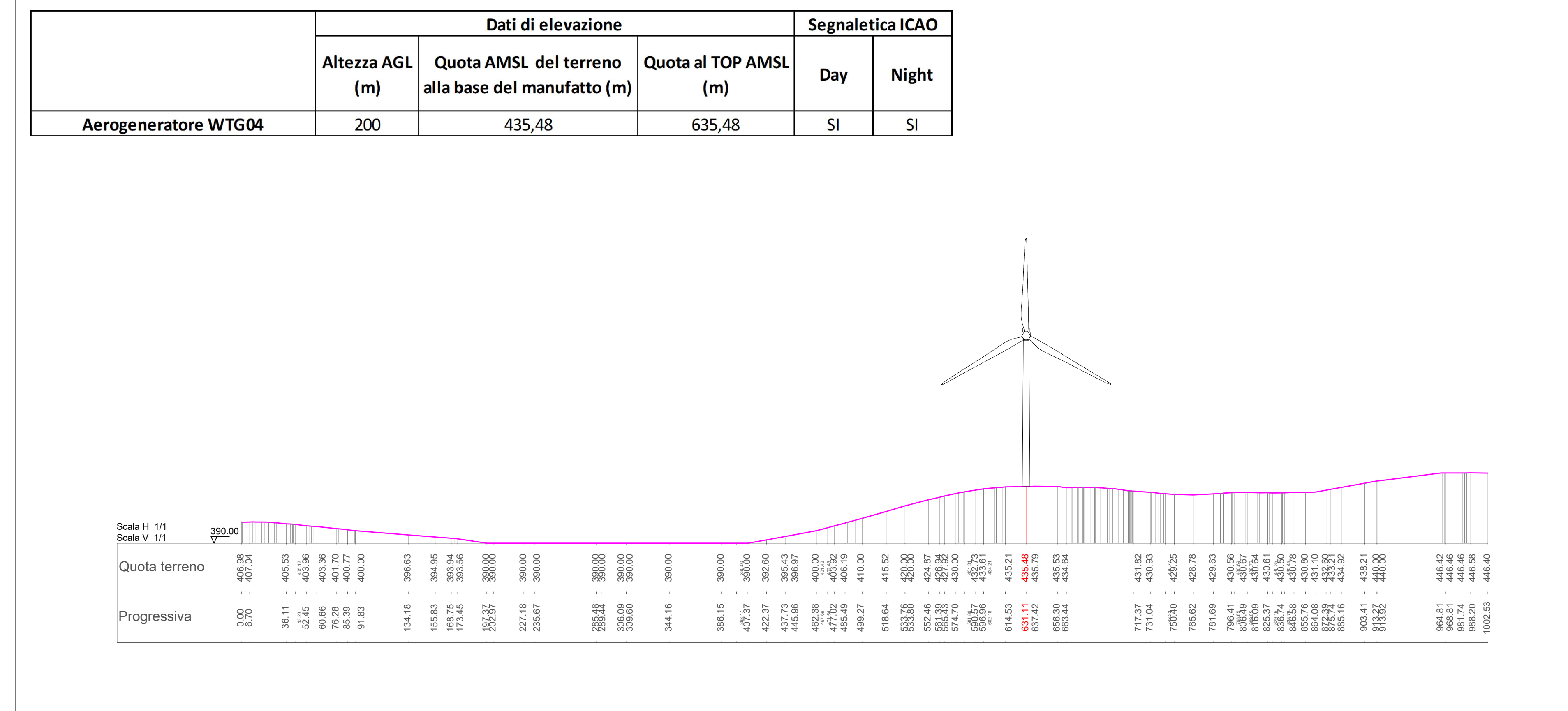
RAPPRESENTAZIONE PROFILO ALTIMETRICO - AEROGENERATORE WTG04 - SCALA 1:2.500
