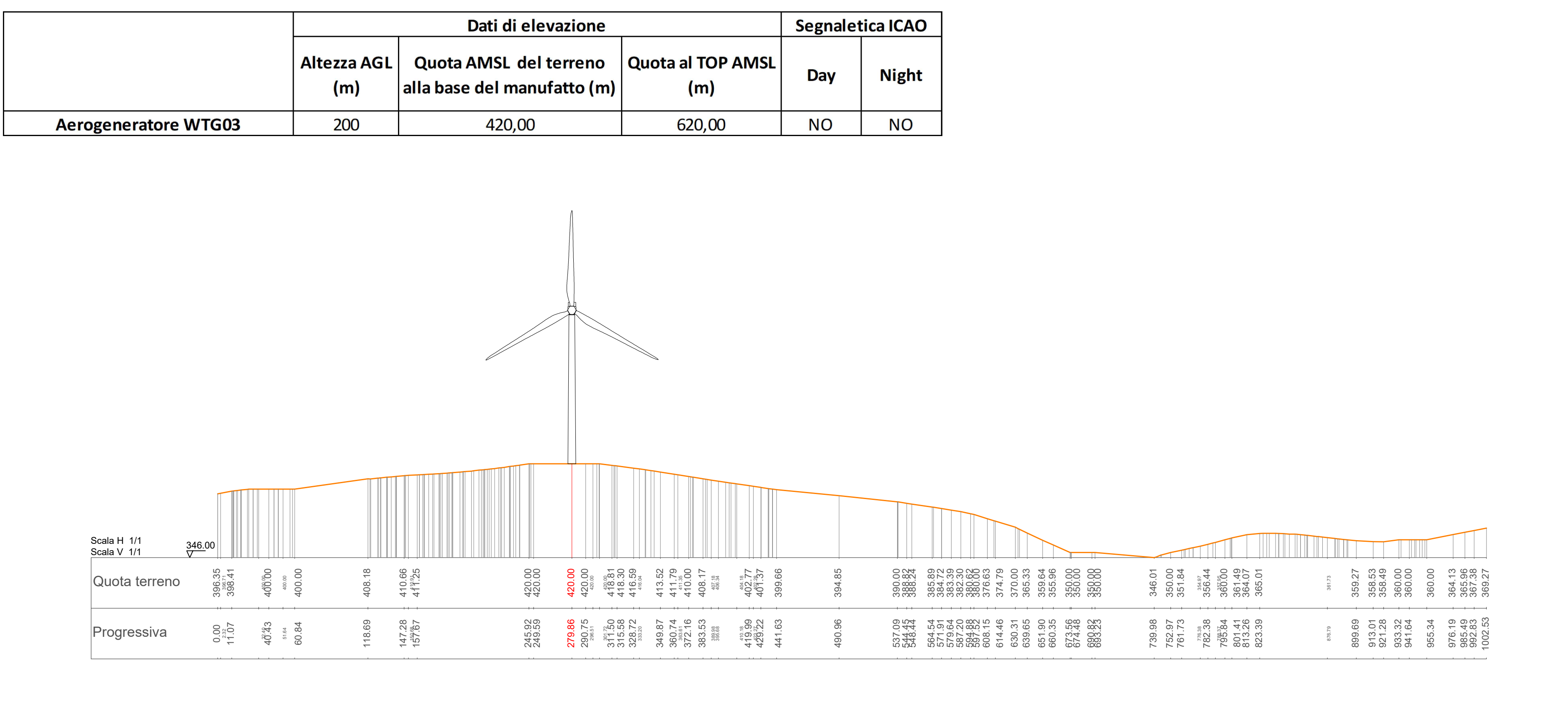
RAPPRESENTAZIONE PROFILO ALTIMETRICO - AEROGENERATORE WTG03 - SCALA 1:2.500
