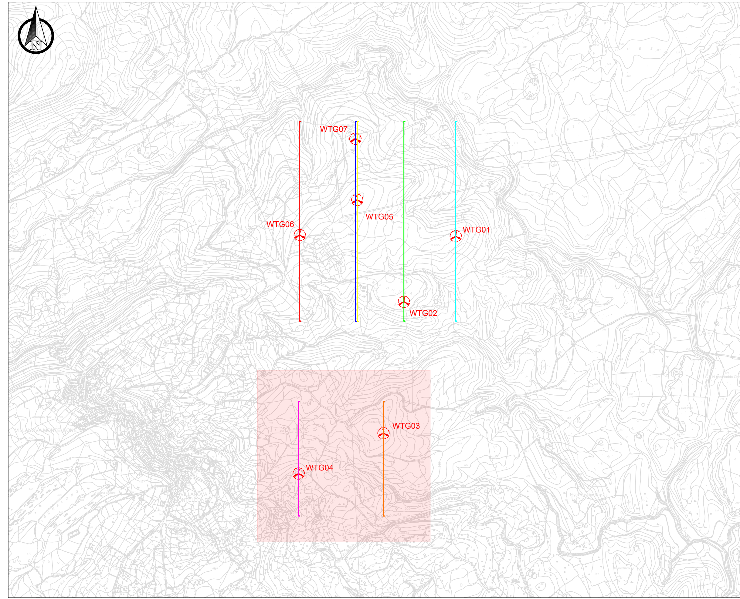
PLANIMETRIA DI INQUADRAMENTO GENERALE - SCALA 1:20.000
