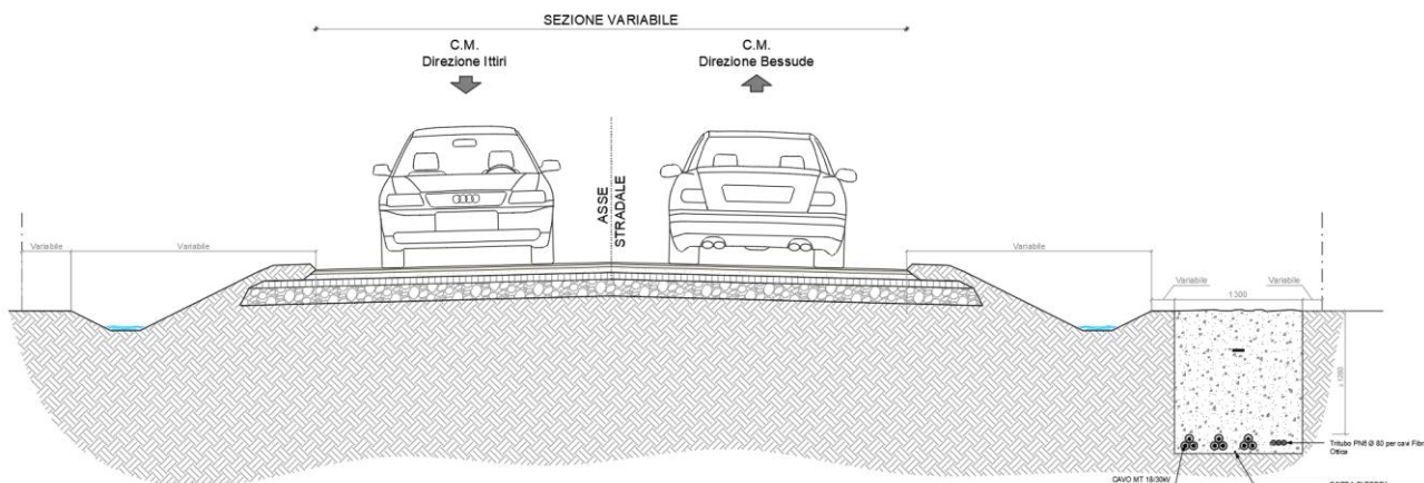
Figura 3.3 - Modalità di posa cavidotto MT in parallelismo strade ANAS
