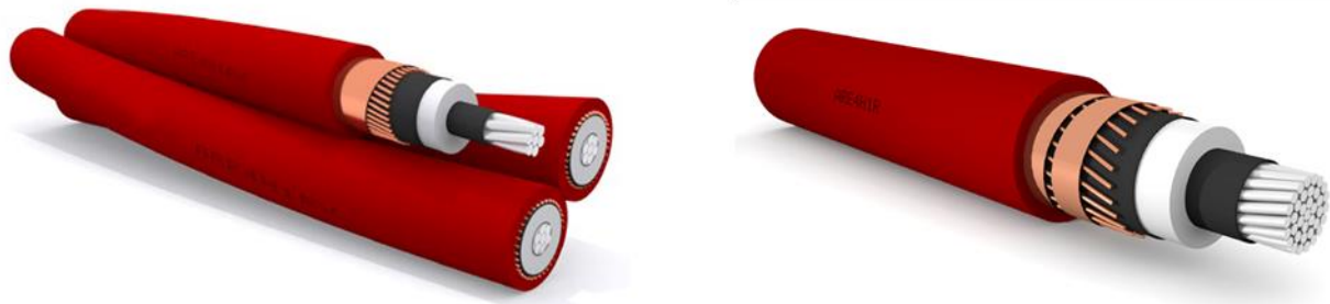
Figura 3.1 - Cavi del tipo ARE4H1RX-18/30 kV e ARE4H1R-18/30 kV
