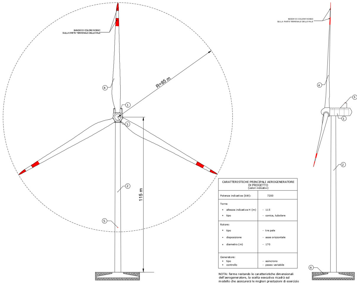
Figura 2.1 – Aerogeneratore di progetto con altezza al mozzo (1) di 115 m e diametro del rotore (3) di 170 m
