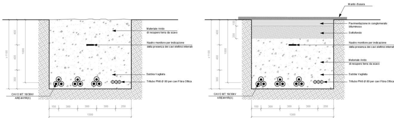
Figura 3.2 – Tipico modalità di posa cavidotto MT
