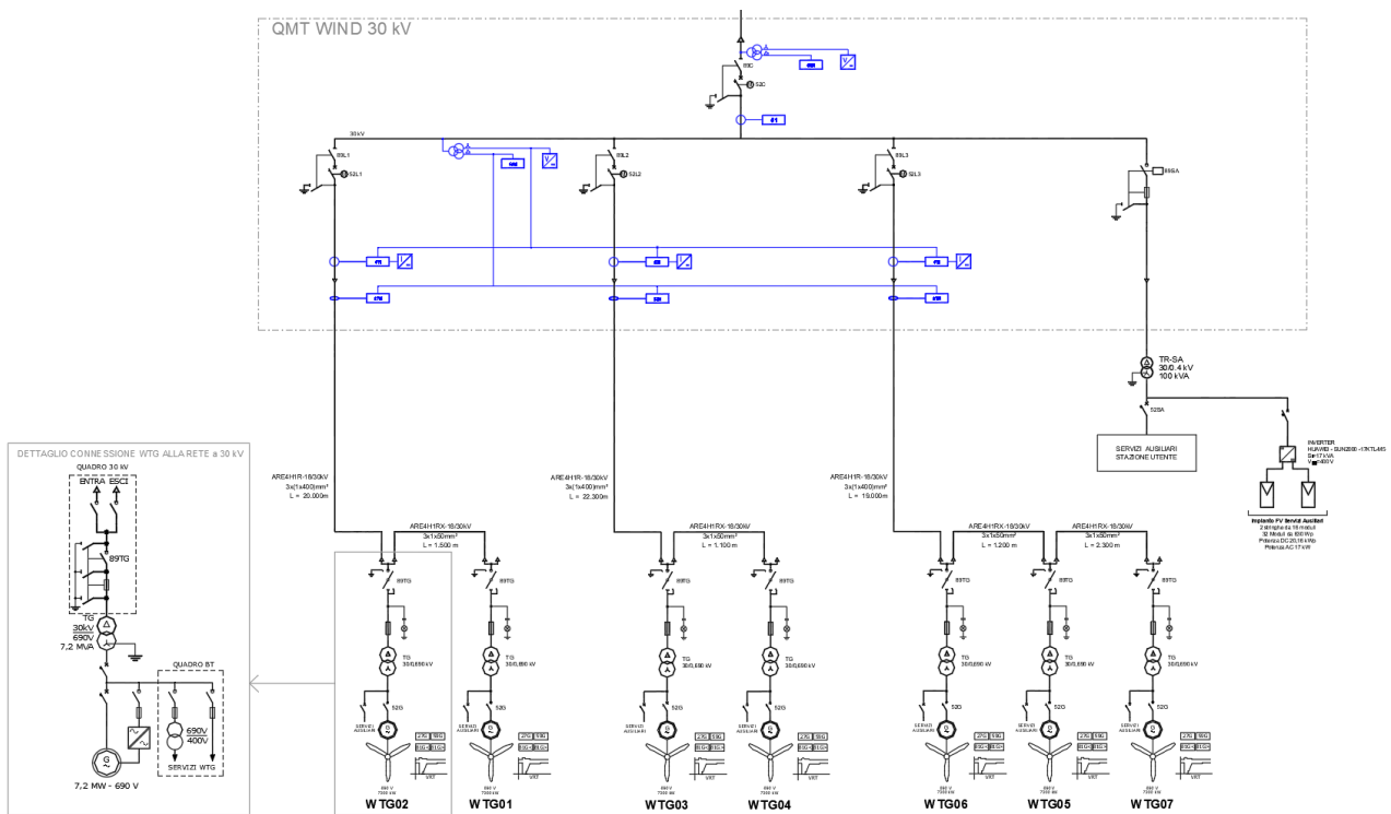
Figura 2.2 – Schema elettrico unifilare impianto di produzione eolica
