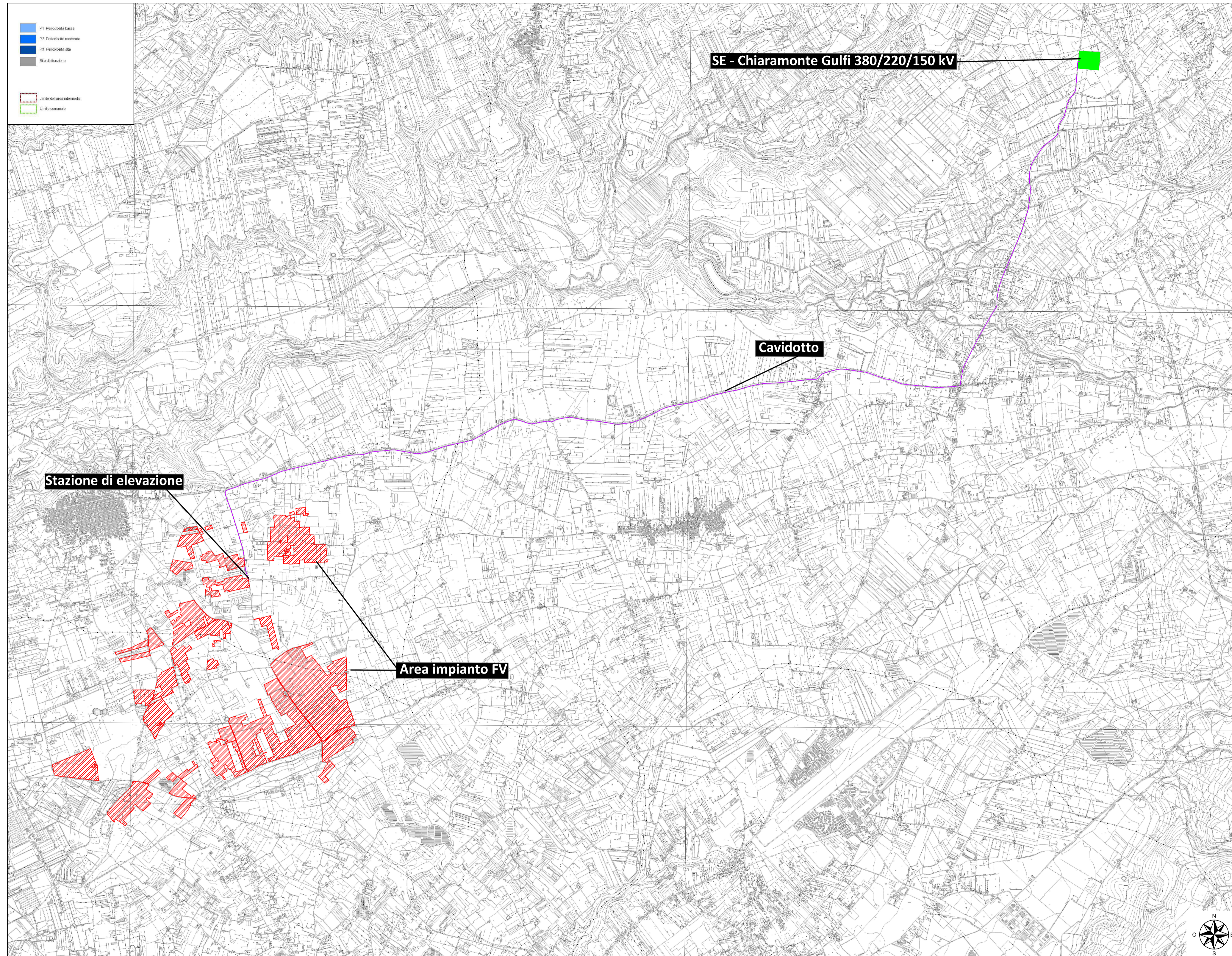
Stralcio "P.A.I." carta della pericolosità idraulica su C.T.R. n° 644100 - 644110 - 644120 - 644140 - 644150 - 644160 - 647020 - 647030 - 647040. Scala 1:30.000
