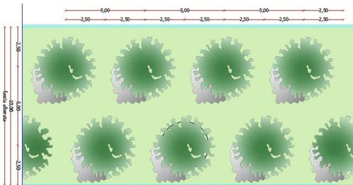
Figura 3 - Schema sintetico sul sesto d'impianto per la fascia arborea di protezione e separazione
