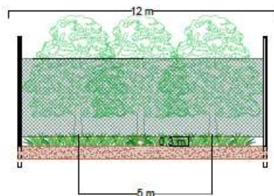
Figura 7 - Esempio di tipologie di sottopassi per la fauna che verranno realizzati
