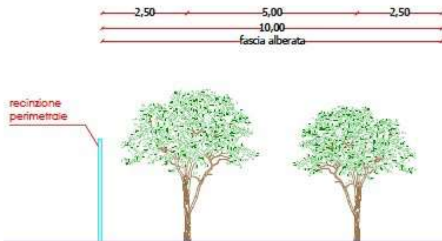
Figura 2 - Sezione fascia arborea di protezione e separazione
