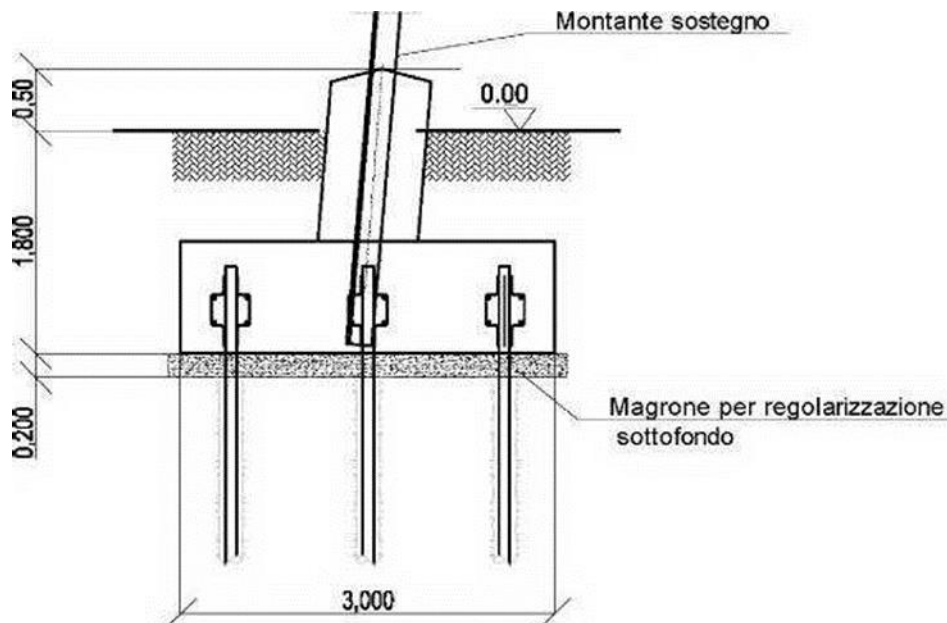
Figura 6 - Disegno costruttivo di un micropalo
