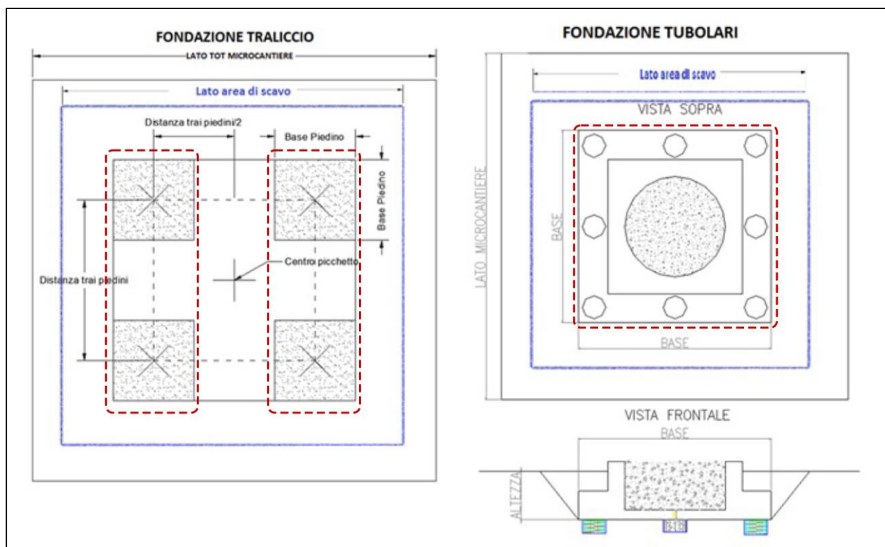
Figura 10 - Schematico di fondazione: i rettangoli rossi indicano il posizionamento dei saggi archeologici
