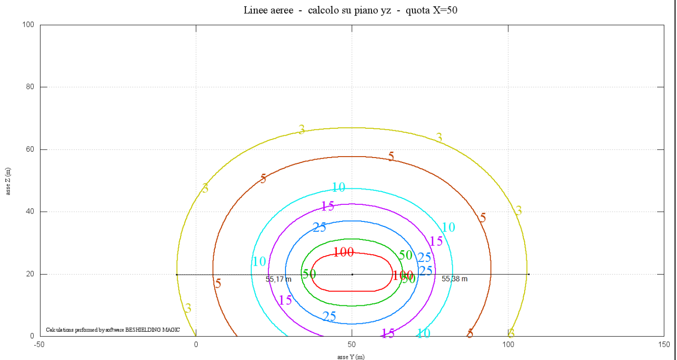
Figura 3 – Livelli di campo magnetico prodotti dalla configurazione dei conduttori su sostegno a Y in rettilifo
