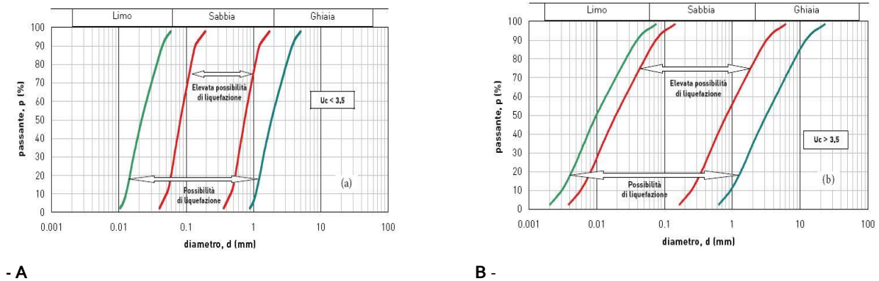
Figura 15 A Fusi granulometrici suscettibili a liquefazione con U < 3.5
