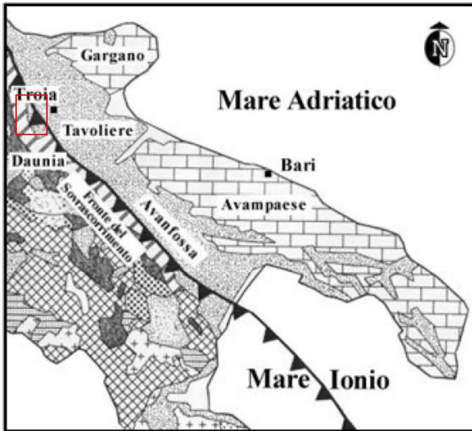
Figura 2 Distinzione dei domini geologici (Bruno G. et alii, 2006).
