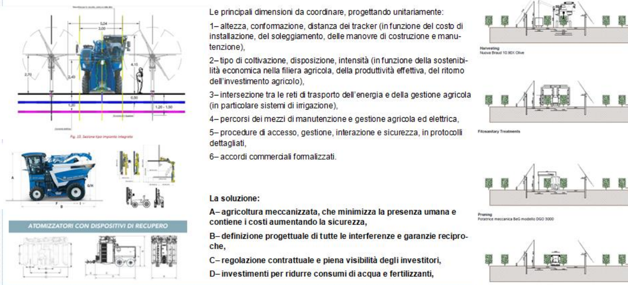
Figura 5 - Concetto agrivoltaico_2
