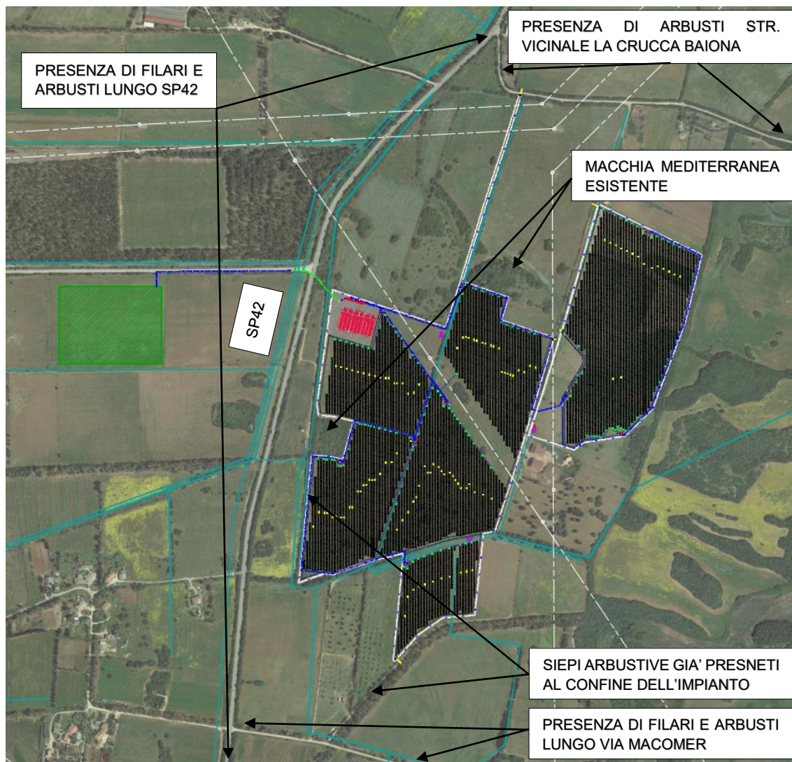
Figura 5 - Planimetria con indicazione della vegetazione di mascheramento
