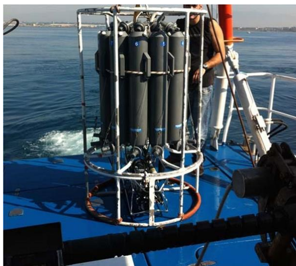
Figura 1.1.3. Sonda multi-parametrica (CTD) SBE 911 plus con multicampionatore d'acqua Carousel SBE 32 con 12 bottiglie Niskin da 10 litri.
