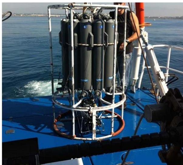
Figura 1.3.3. Sonda multi-parametrica (CTD) SBE 911 plus con multicampionatore d'acqua Carousel SBE 32 con 12 bottiglie Niskin da 10 litri.
