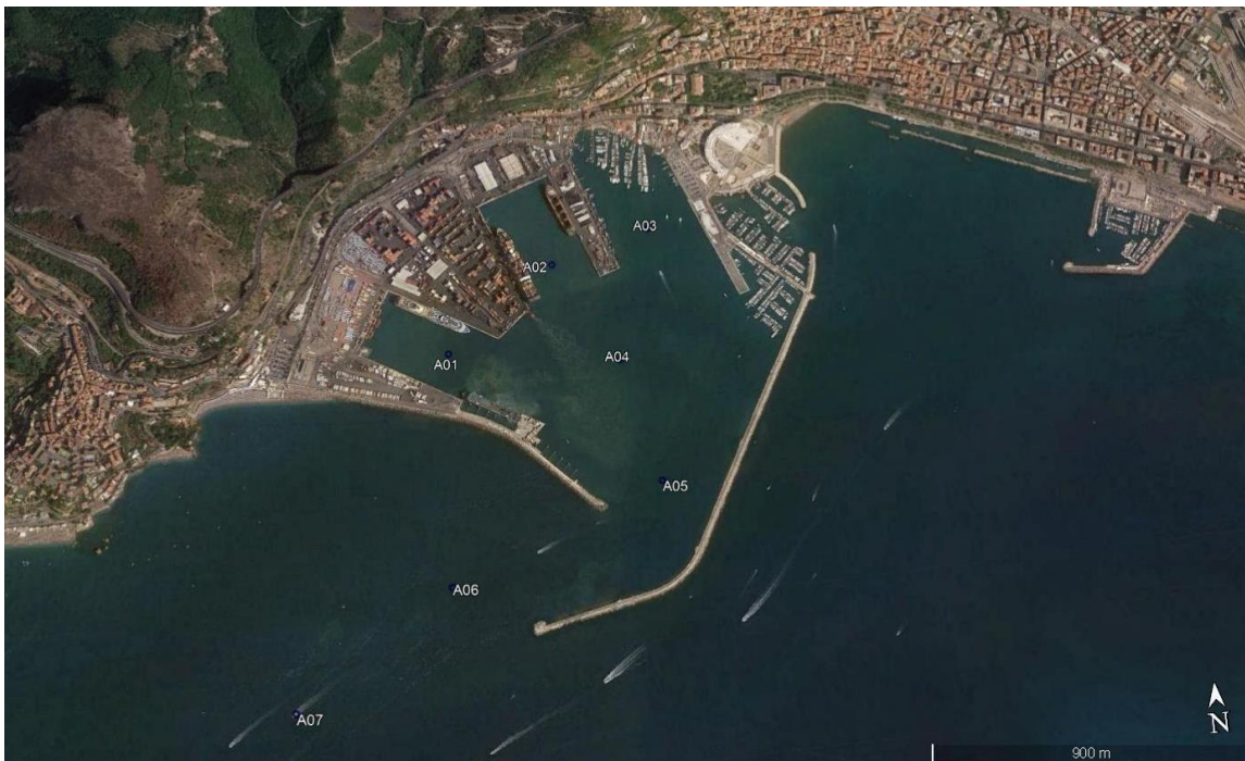
Figura 1.1.1. Ubicazione delle stazioni di campionamento (colonna d’acqua).
