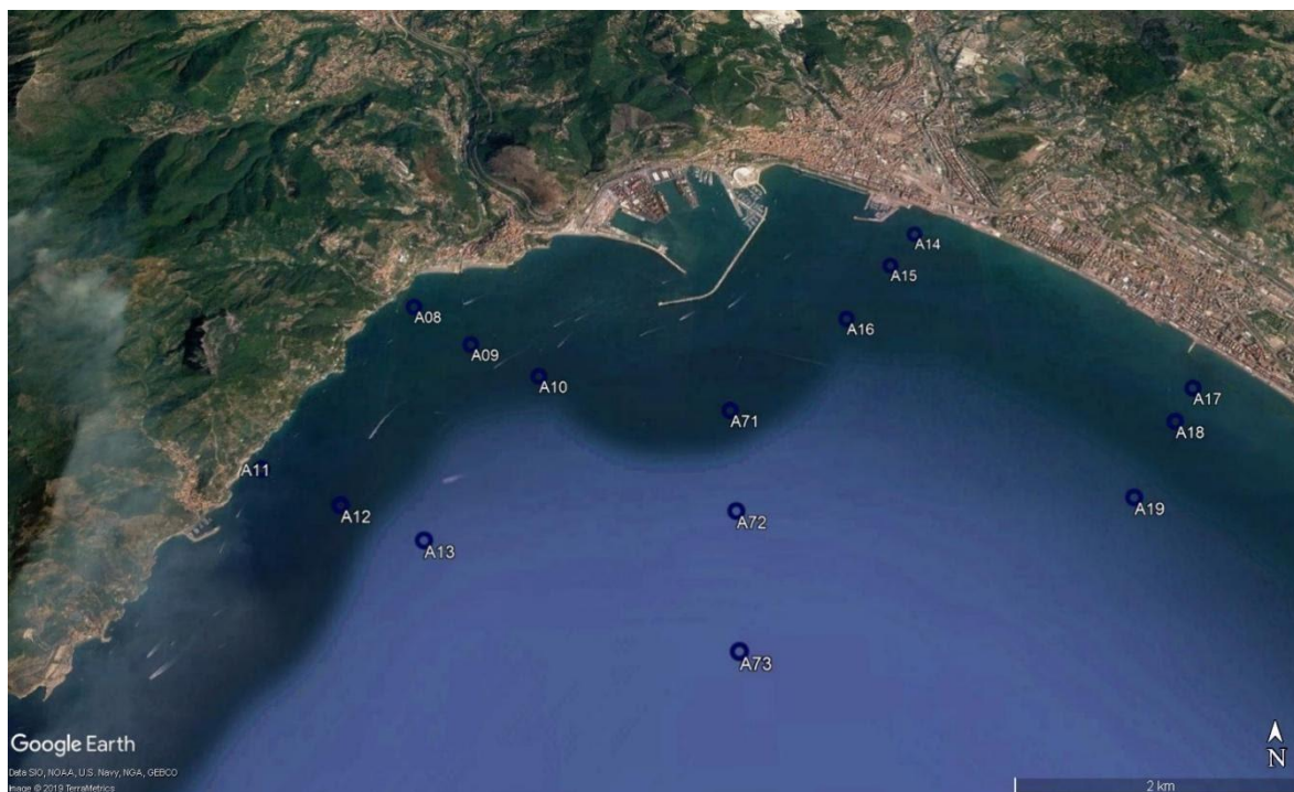
Figura 1.2.1. Ubicazione delle stazioni di campionamento (colonna d'acqua).
