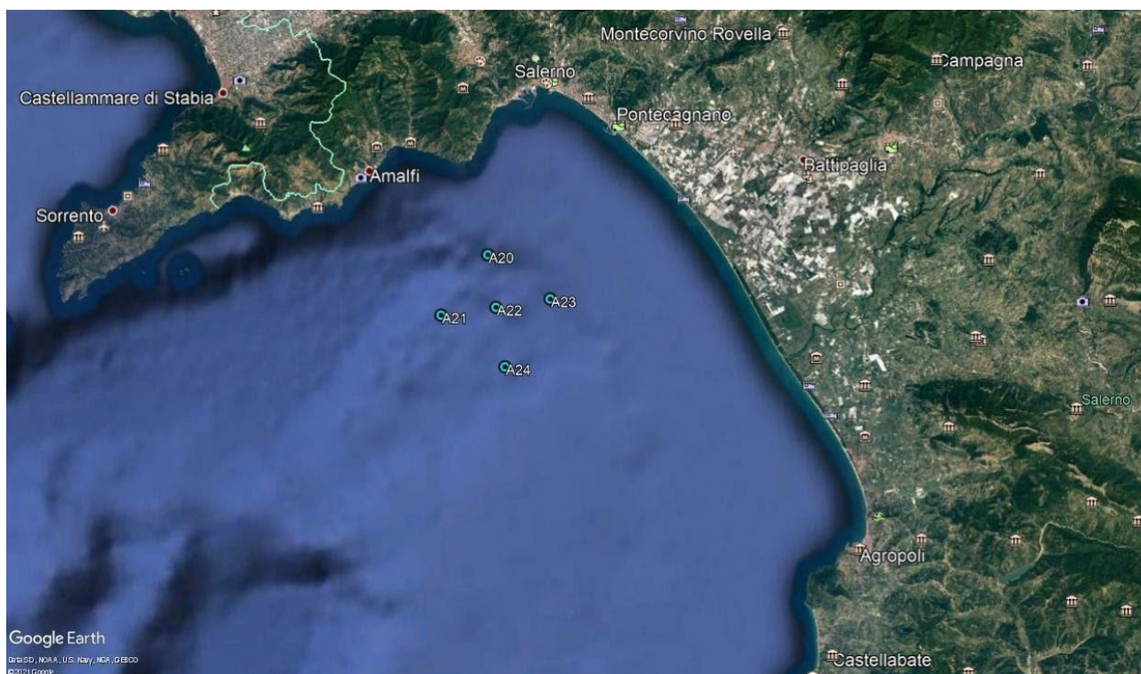
Figura 1.3.1. Ubicazione delle stazioni di campionamento (colonna d'acqua).
