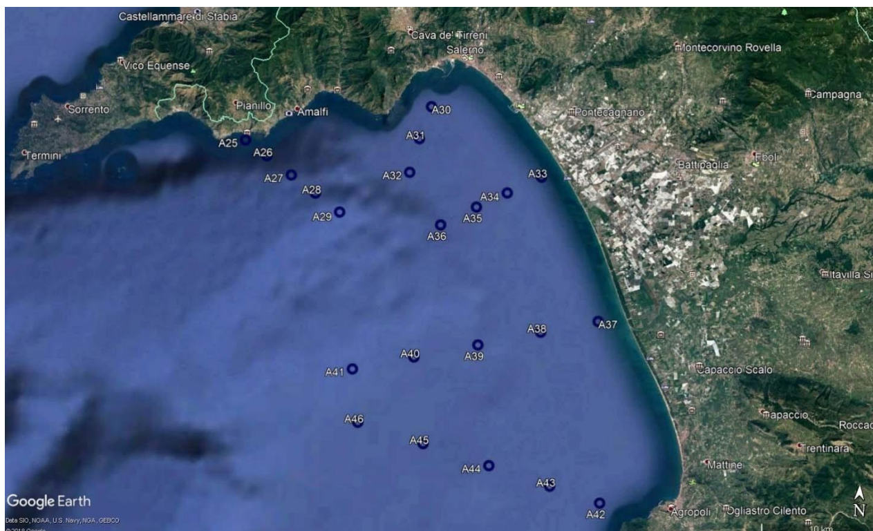
Figura 1.4.1. Ubicazione delle stazioni di campionamento (colonna d'acqua).
