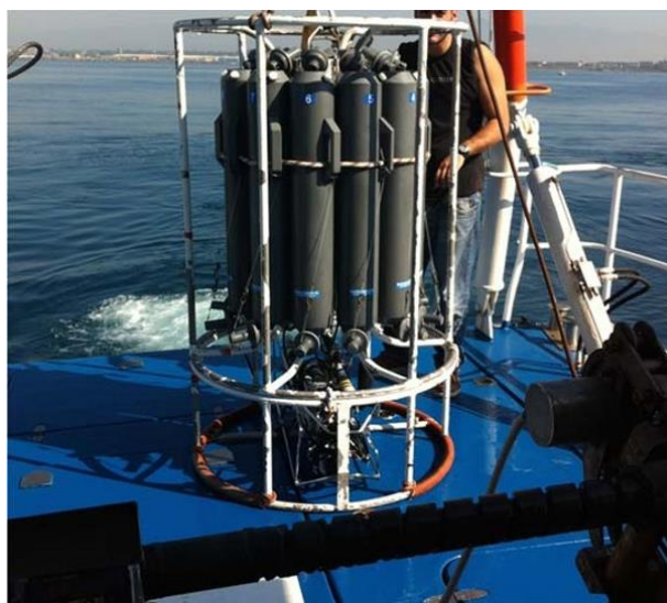
Figura 1.5.3. Sonda multi-parametrica (CTD) SBE 911 plus con multicampionatore di acqua Carousel SBE 32 con 12 bottiglie Niskin e da 10 litri.
