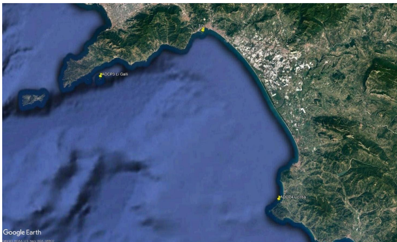
Figura 3.2. Ubicazione geografica delle stazioni di monitoraggio.
