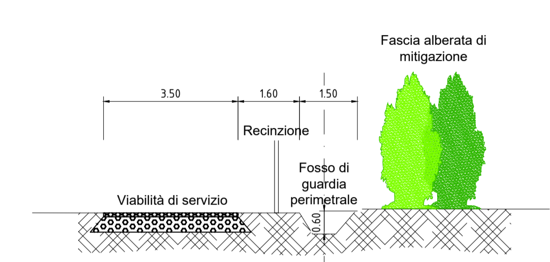
SEZIONE TIPICA DI VIABILITA' PERIMETRALE E FOSCO DI GUARDIA DI PROGETTO 1:100
