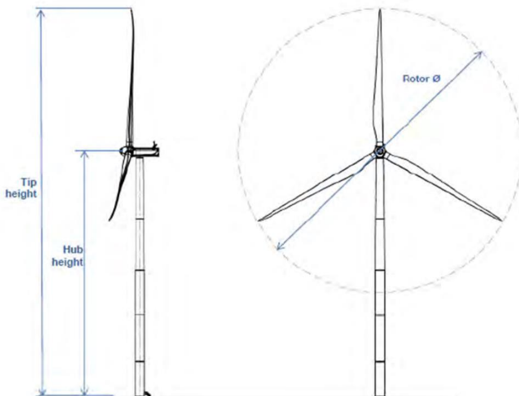
Figura 15: Dimensioni aerogeneratori da 6.6 MW in progetto
