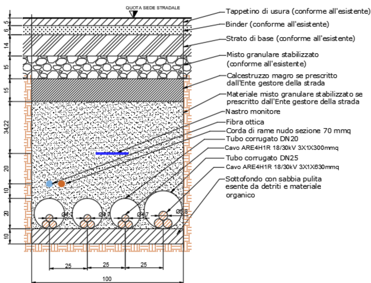
Figura 2 – Sezione cavidotto MT dell'impianto di S. Antonio di Gallura: quattro terne di cavi a 30 kV su strada asfaltata
