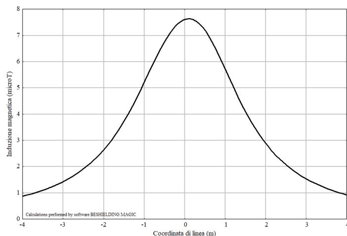
Figura 4 – Valori di induzione magnetica sul livello stradale del cavidotto MT dell’impianto di S. Antonio di Gallura formato da quattro terne di cavi a 30kV
