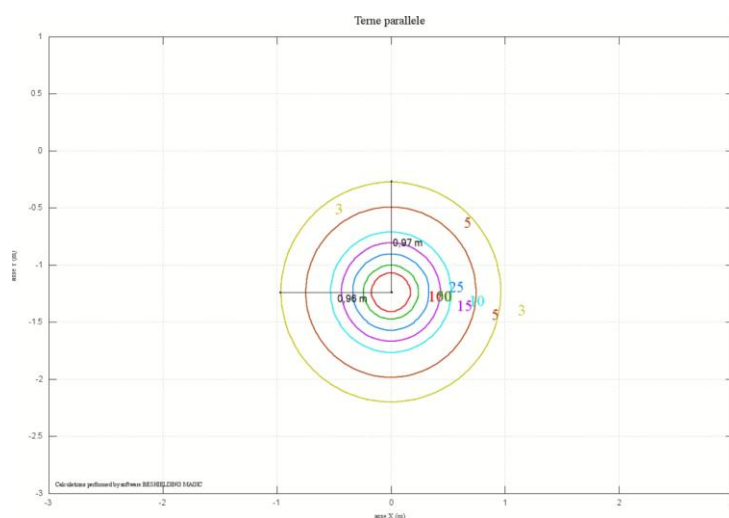
Figura 6 Curve di isolivello – simulazione cavidotto MT dell'impianto BESS di S, Antonio di Gallura
