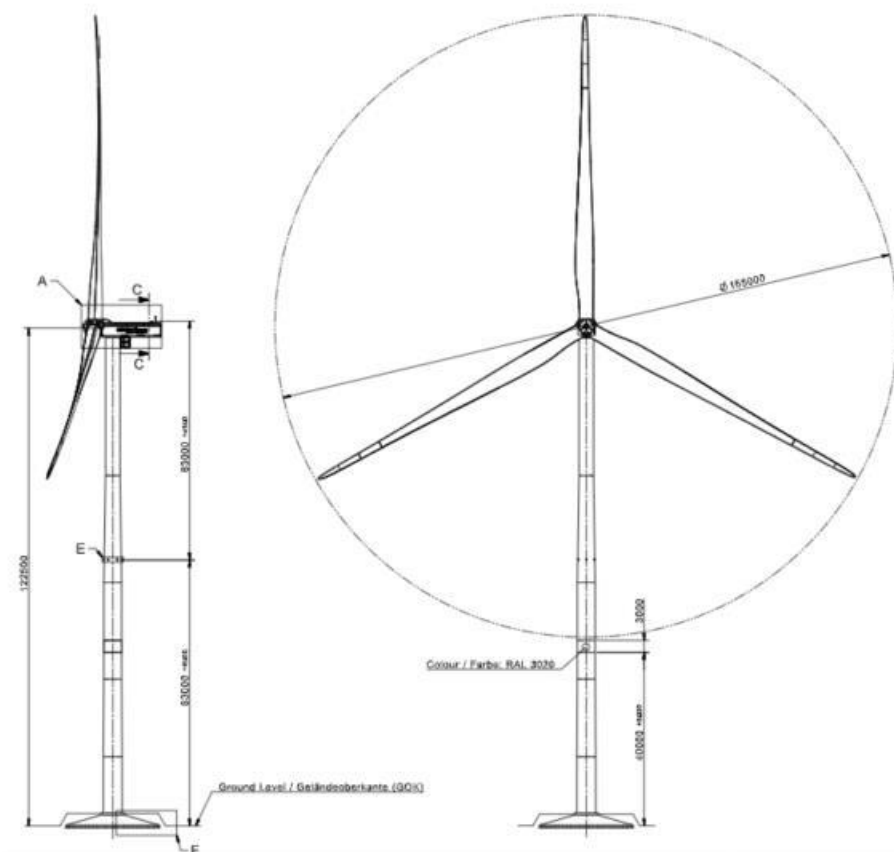
Figura 2: Dimensioni aerogeneratore tipo
