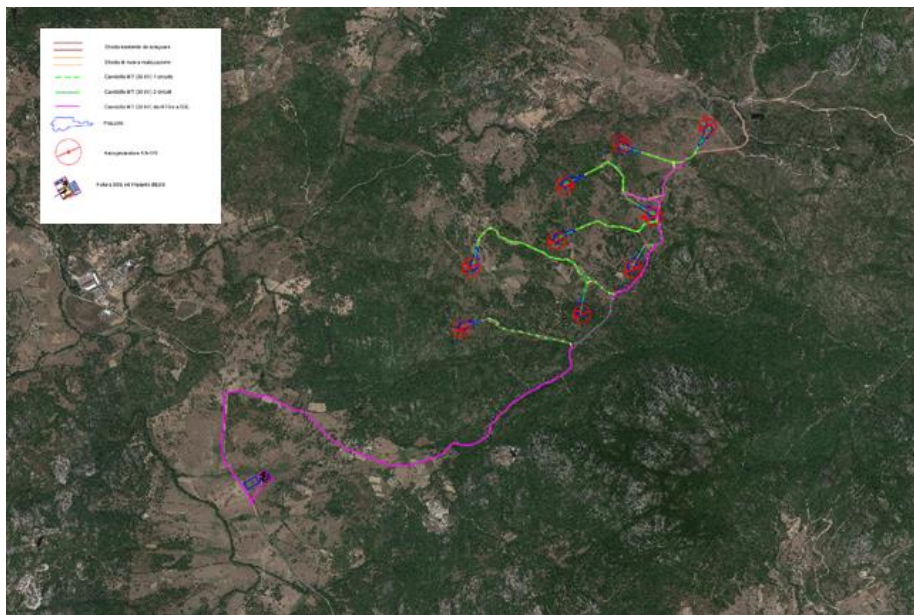
Figura 1 - Primo inquadramento dell'ubicazione delle WTG, della viabilità di impianto e del Cavidotto MT 30 kV su base ortofoto
