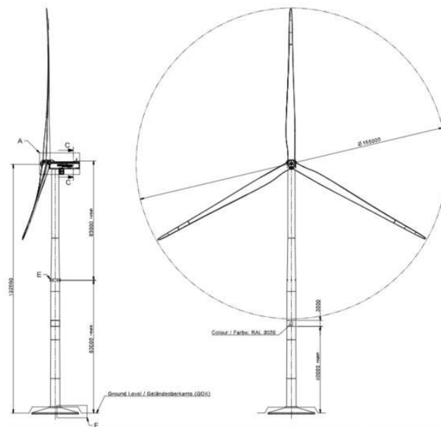
Figura 2 Dimensioni aerogeneratore tipo
