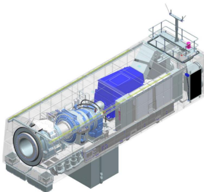
Figura 3 Allestimento navicella dell'aerogeneratore
