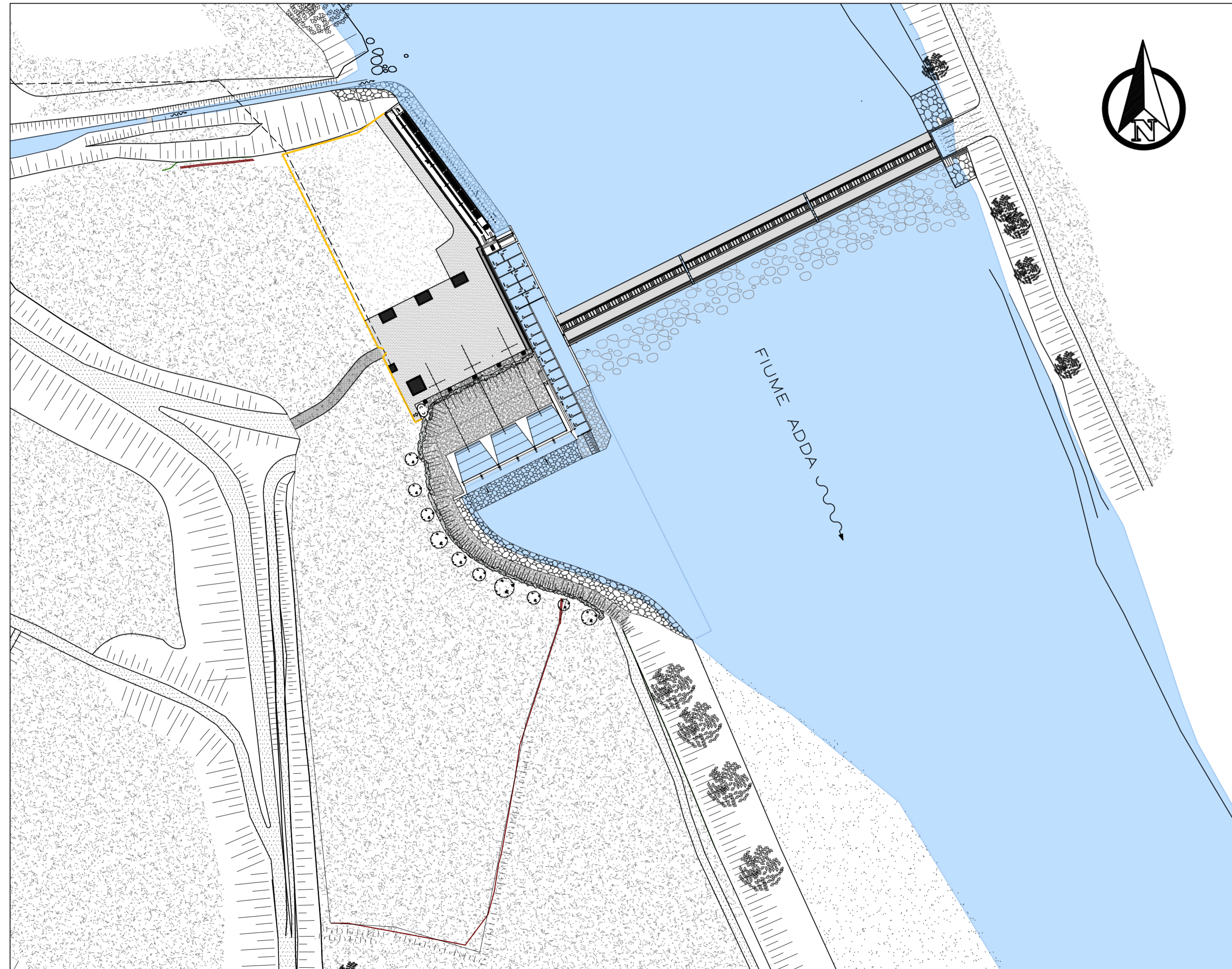
PLANIMETRIA DI PROGETTO 1:1.000
