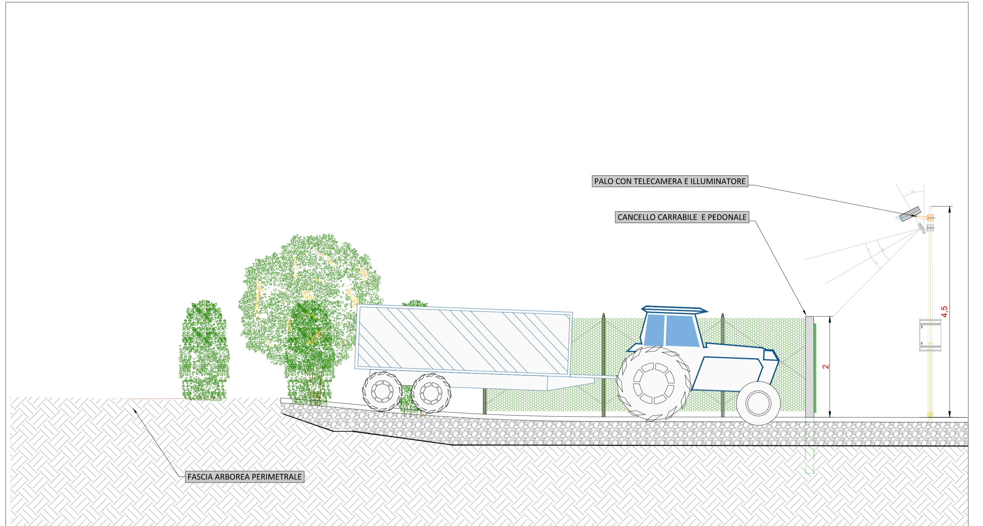
Sezione trasversale - Scala 1:50
