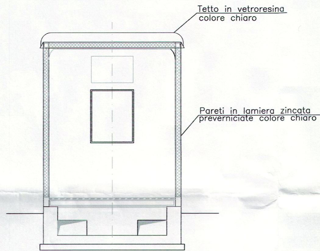
SEZIONE W-W
