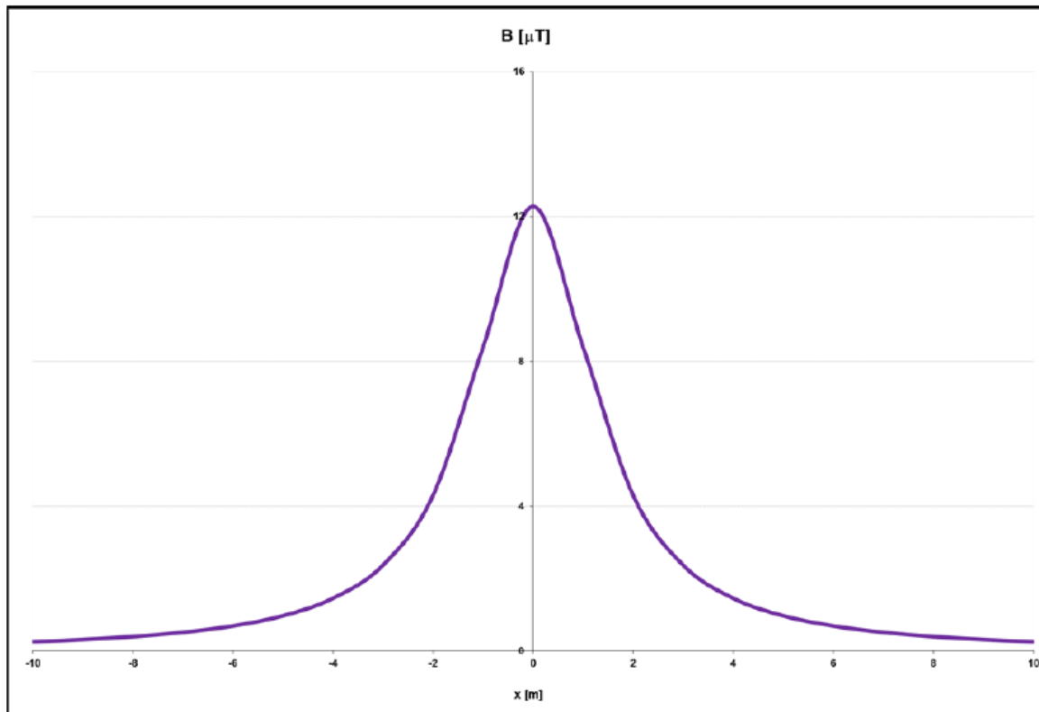
Figura 12: induzione magnetica generata durante l'esercizio dalla linea valutata applicando la procedura delle Norme CEI 211-4 – Guida ai metodi di calcolo dei campi elettrici e magnetici generati da linee elettriche
