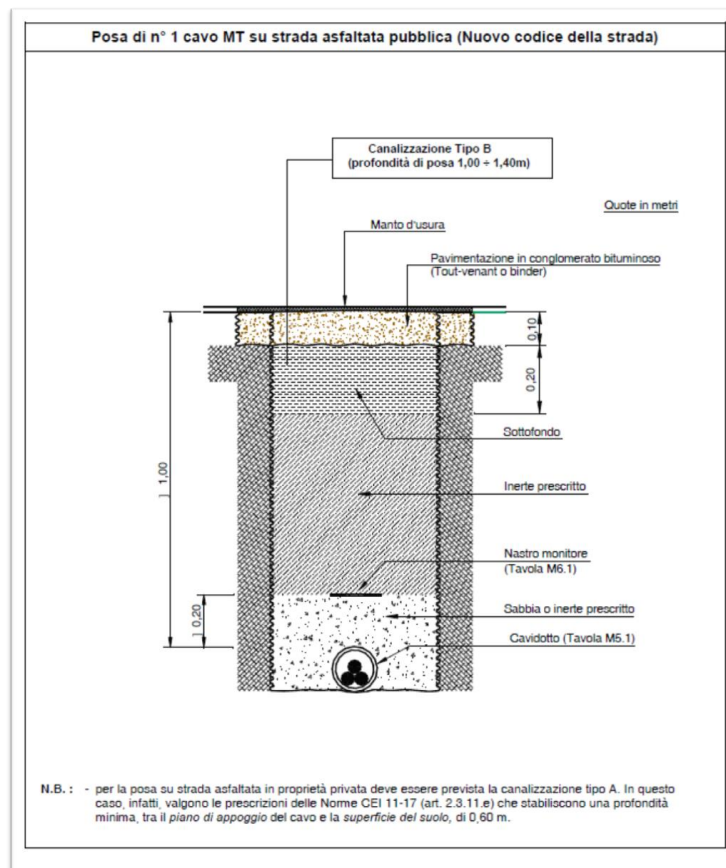
Figura 12: posa indiretta cavi su strada pubblica
