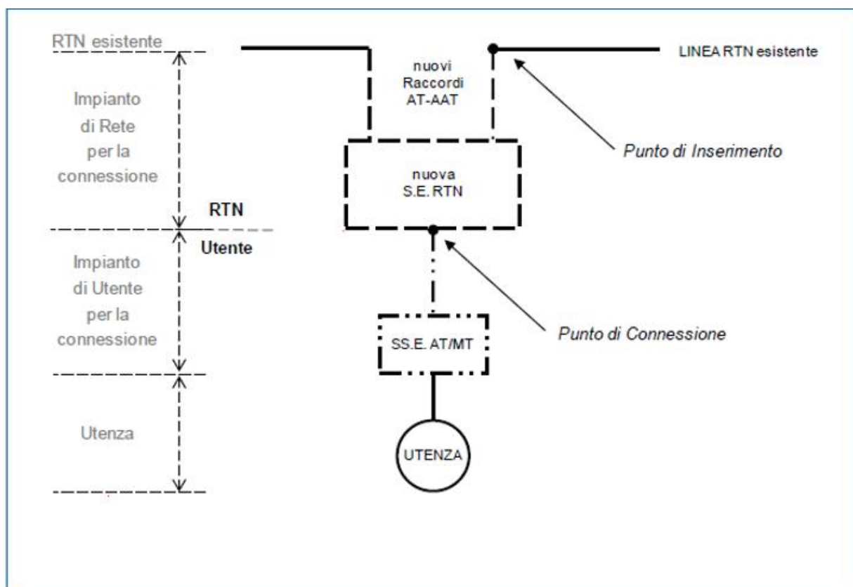
Figura 1: schema tipico di inserimento in antenna su nuova SE RTN
