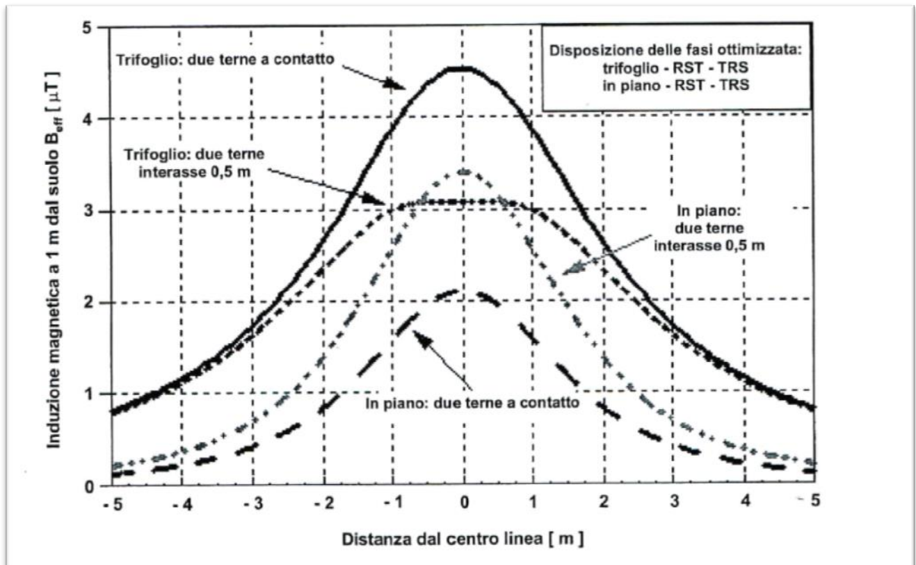
Figura 17: confronto tra livelli di campo magnetico generato dalle linee elettriche interrate in doppia terna
