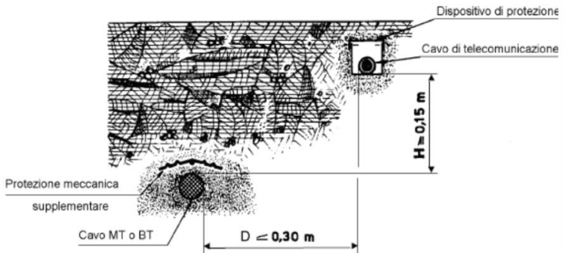
Figura 4: provvedimenti da adottare in caso di interferenze con cavi di telecomunicazione caso a)
