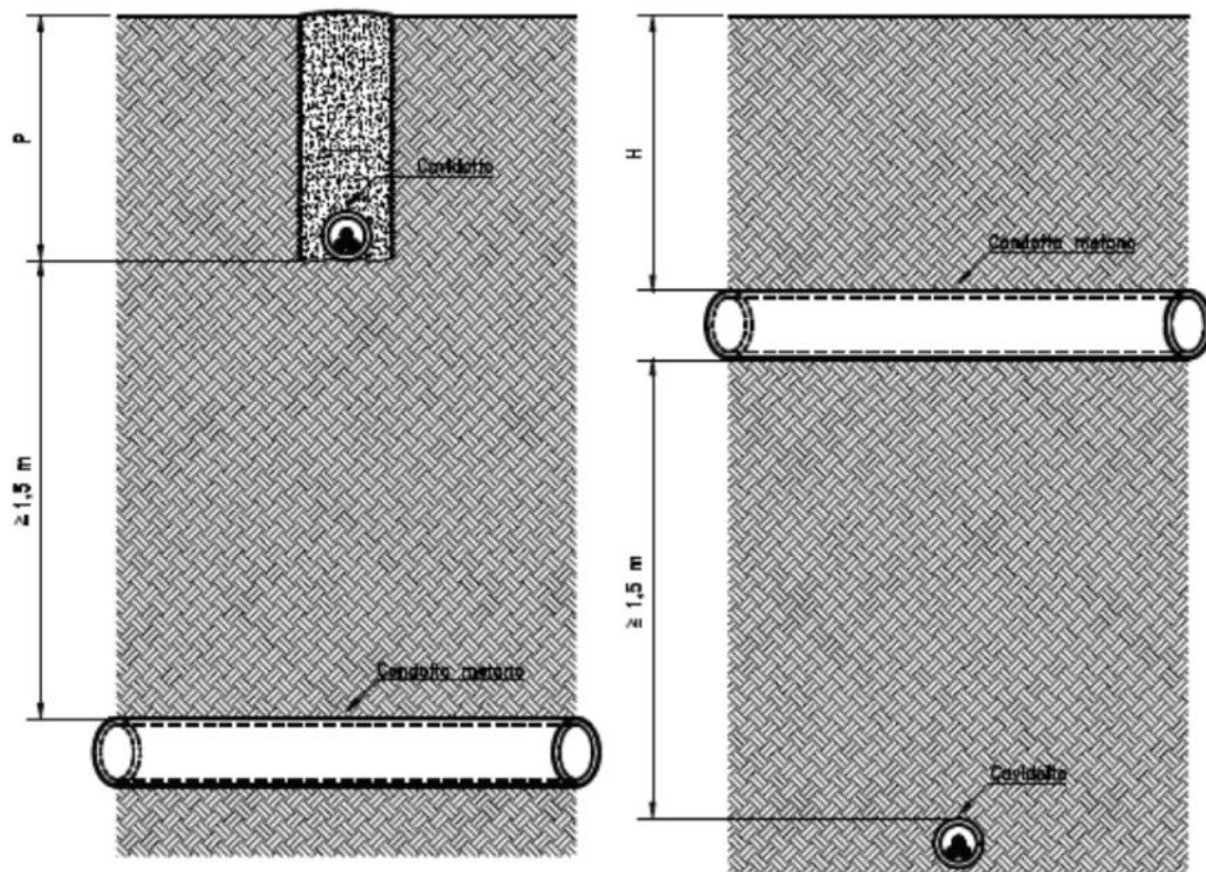
Figura 10: provvedimenti da adottare in caso di interferenze con tubazioni metalliche caso d)
