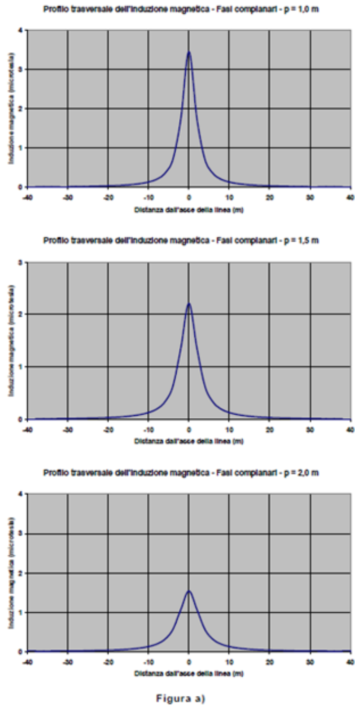
Figura 15: Figura a) tratta dalla Norma CEI 11-17
