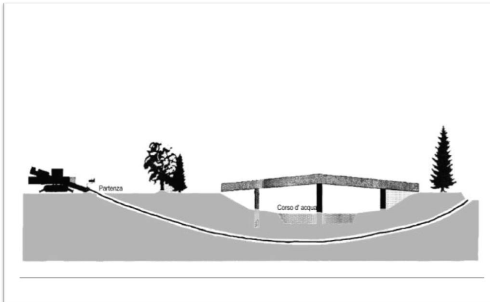
Figura 11: esempio tipico di trivellazione orizzontale controllata
