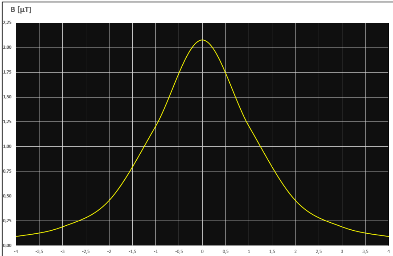
Figura 18: Induzione Magnetica generata dalla dorsale 36 kV
