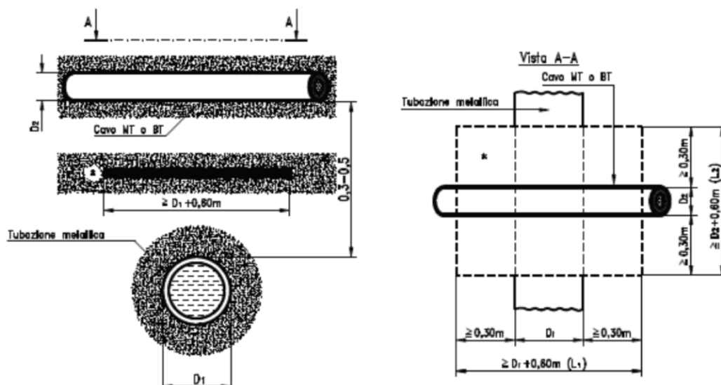
Figura 7: provvedimenti da adottare in caso di interferenze con tubazioni metalliche caso a)
