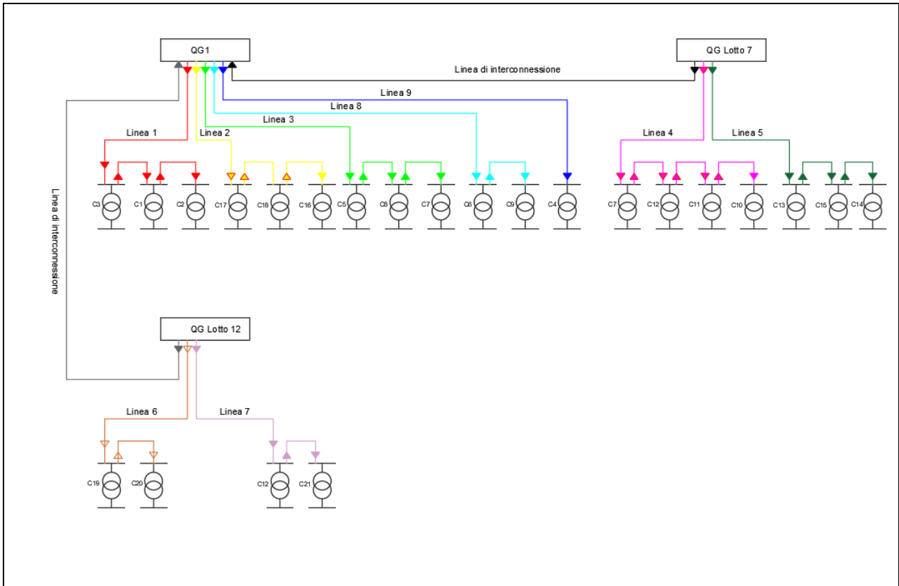
Figura 2: schema a blocchi impianto
