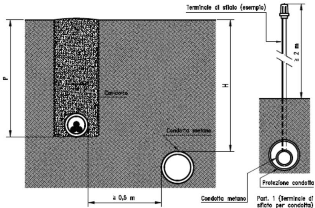
Figura 9: provvedimenti da adottare in caso di interferenze con tubazioni metalliche caso c)
