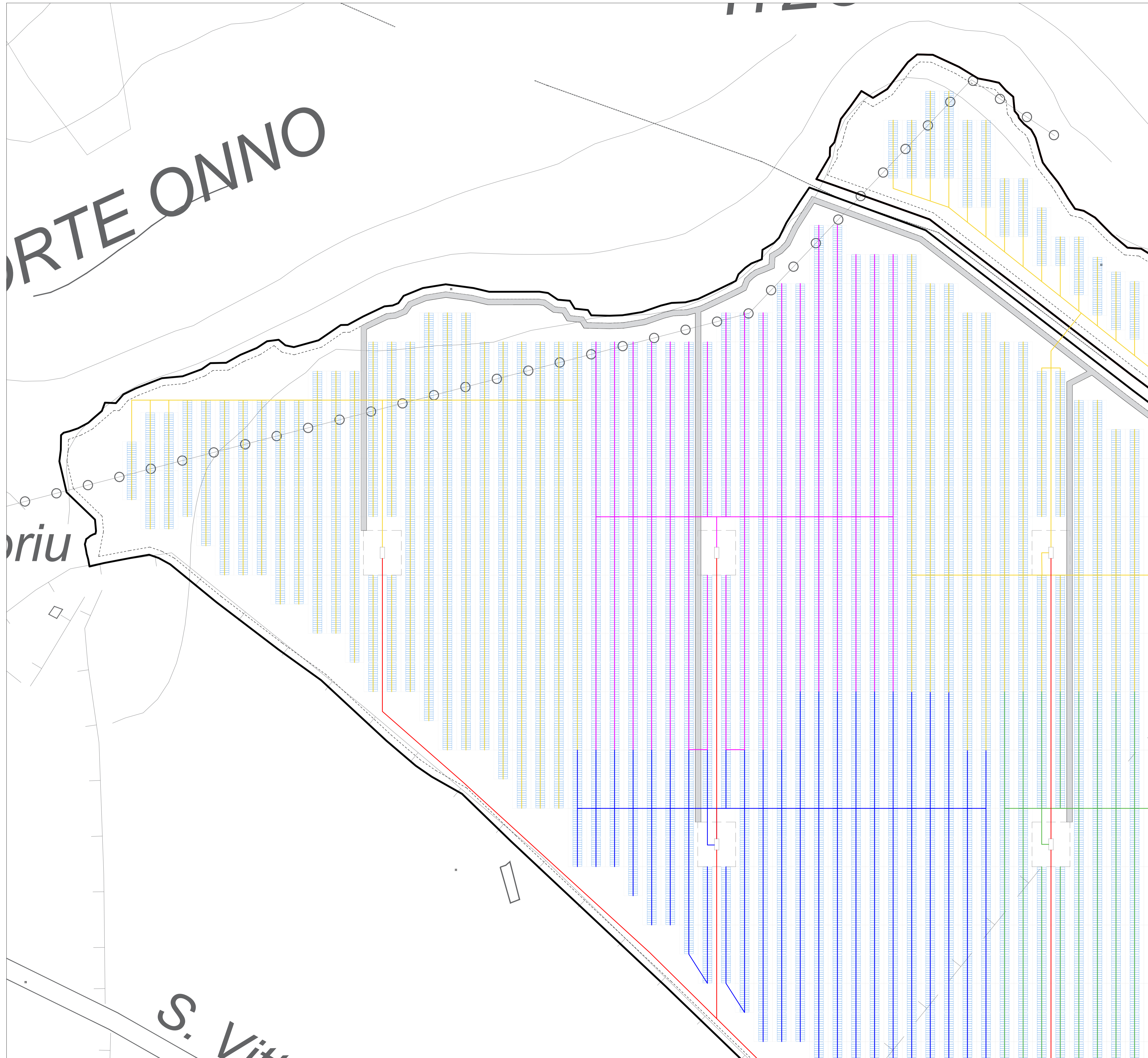
PLANIMETRIA CAVIDOTTI IMPIANTO AGRIVOLTAICO - SEZIONE 1
