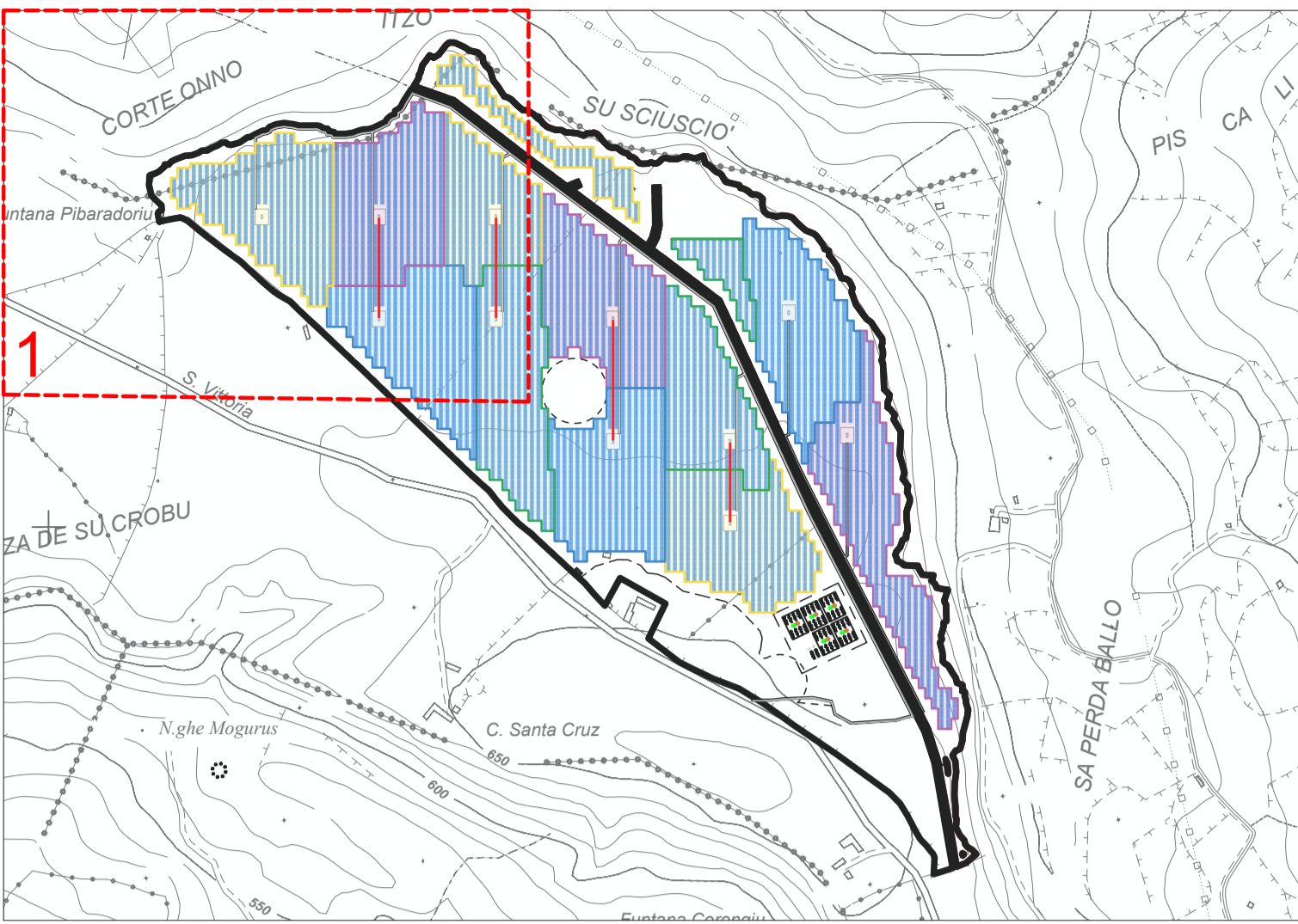
Suddivisione in sezioni - impianto agrivoltaico
