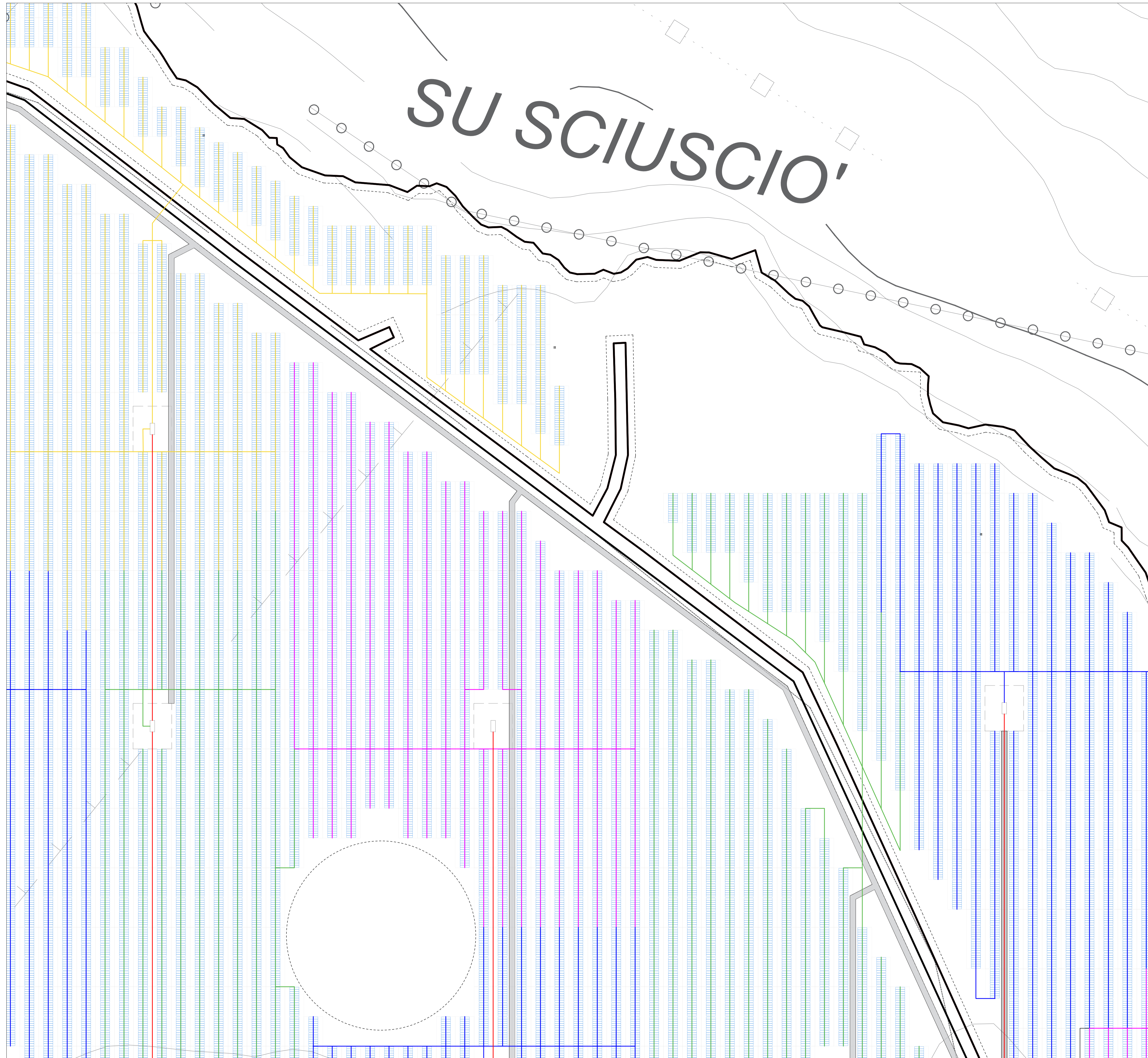
PLANIMETRIA CAVIDOTTI IMPIANTO AGRIVOLTAICO - SEZIONE 2
