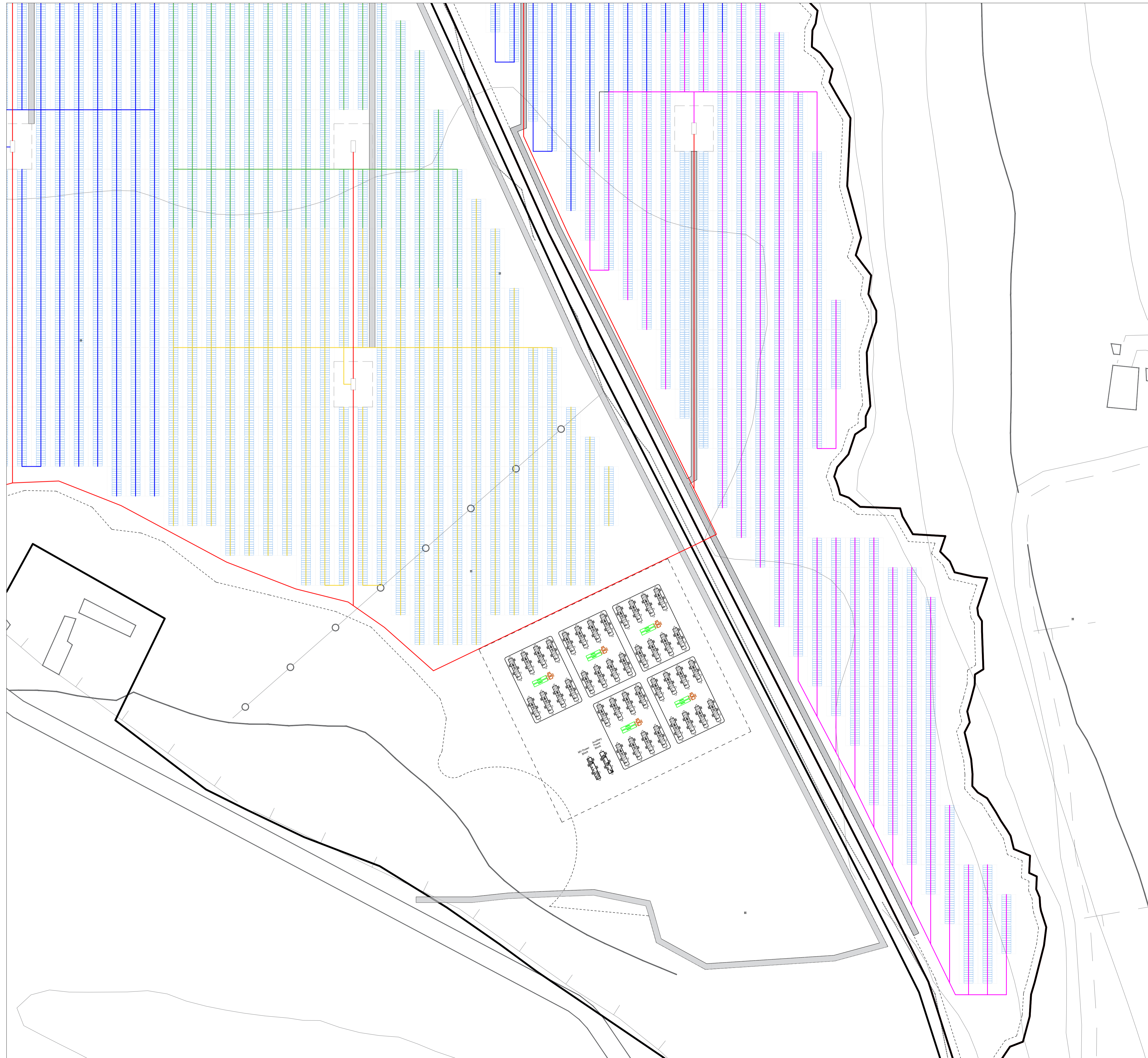
PLANIMETRIA CAVIDOTTI IMPIANTO AGRIVOLTAICO - SEZIONE 4
