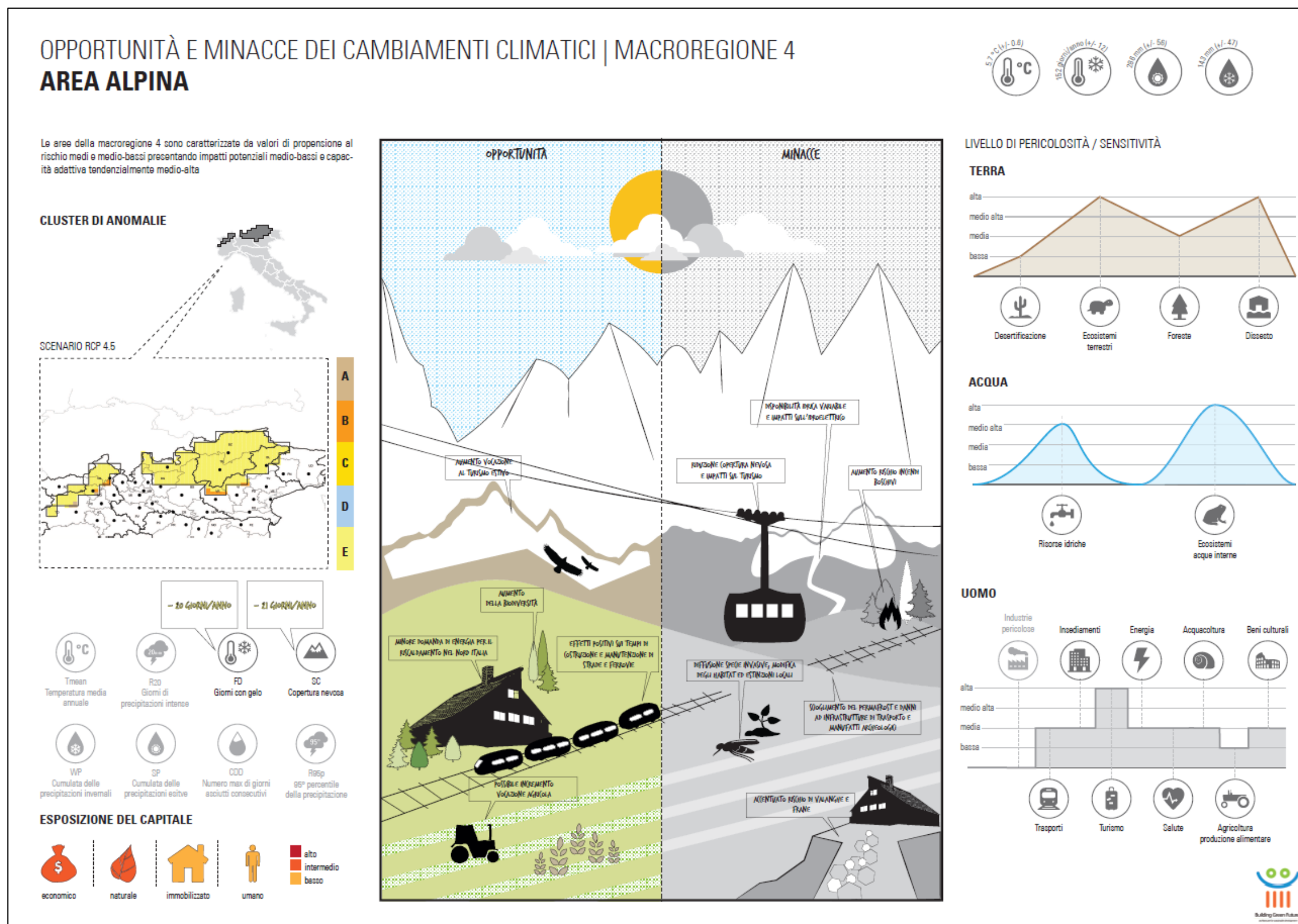
Figura 2 - Infografica degli impatti del cambiamento climatico sulla macroregione 4 – Area alpina
