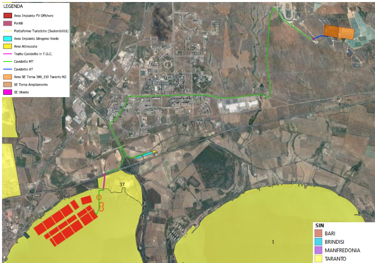
Figura 4-1: Inquadramento territoriale dell'impianto su Ortofoto in Area SIN
