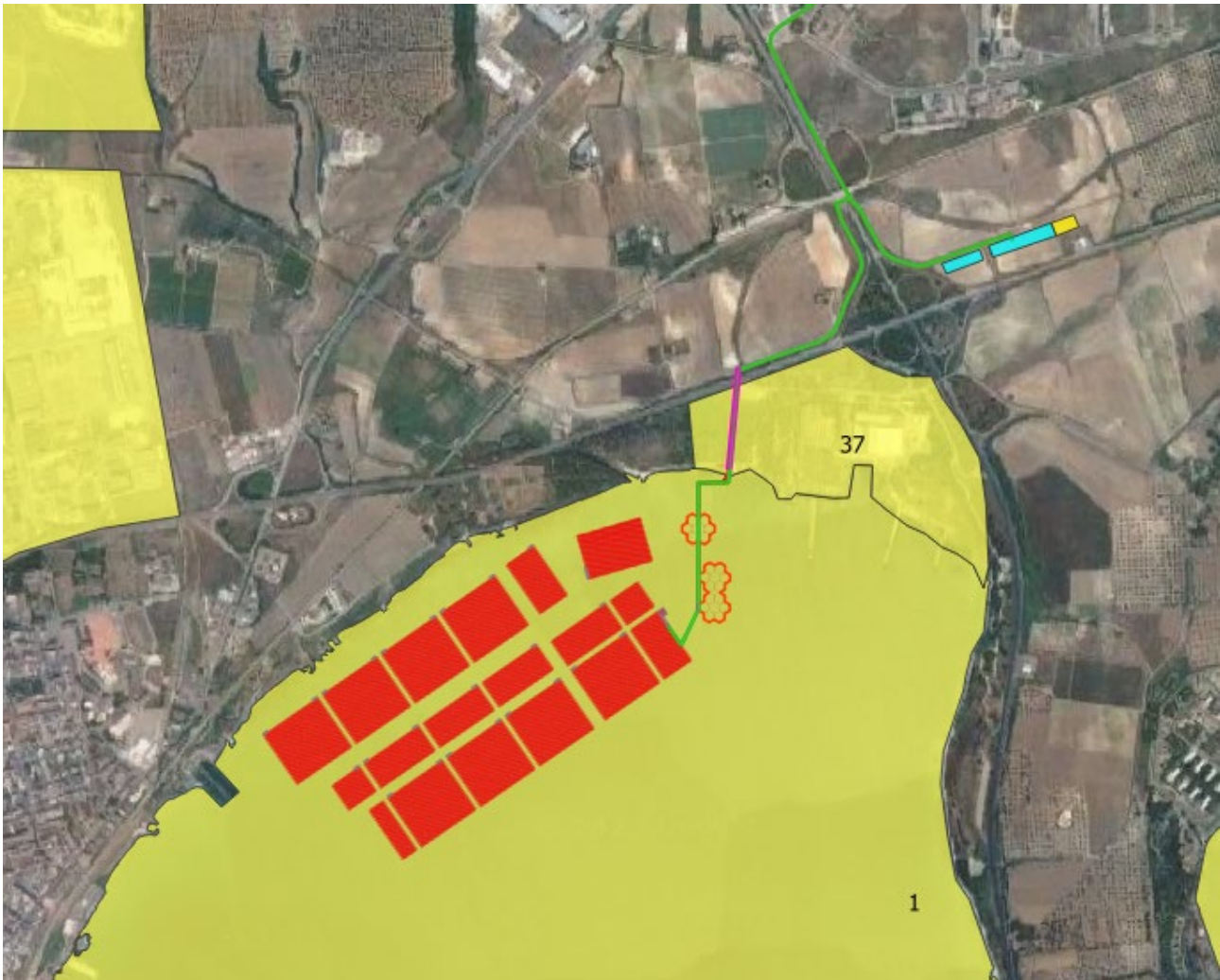
Figura 5-3: Interventi di installazione fotovoltaico in area SIN di Taranto: Particolare area di progetto FV
