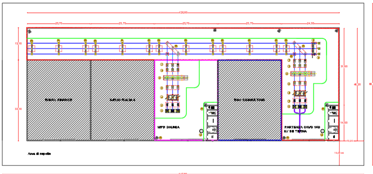
Figura 1: Planimetria elettromeccanica SE condivisa 150 kV (perimetrata in rosso a forma di "L") e sottostazione utente WPD Daunia (perimetrata in magenta)
