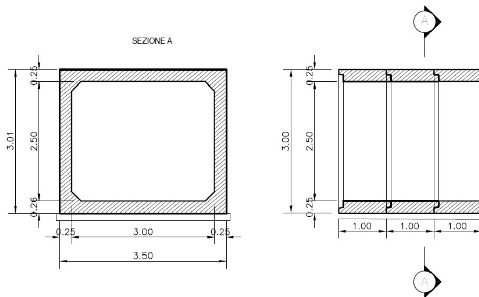
Figura 2 - Sezione dell'opera
