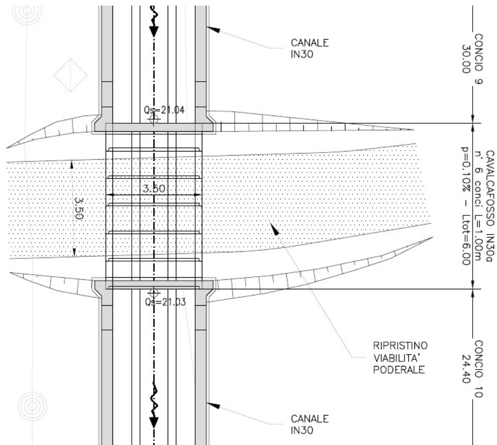
Figura 1 - Pianta tombino
