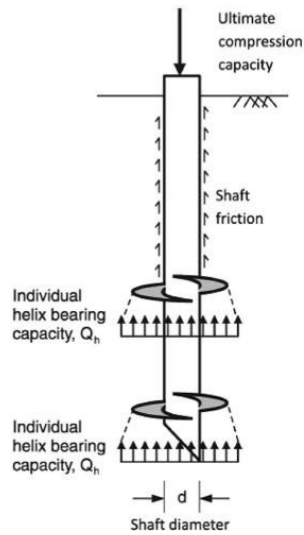
Figura 14 - Metodo della capacità portante individuale Didascalìa Immagini
