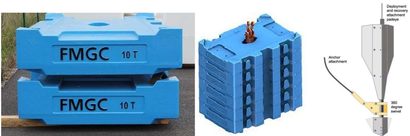
Figura 6 - Illustrazione di ancora a gravità con piastre modulari di ghisa impilate a sinistra. Ancora a gravità con inflessione dinamica a destra.
