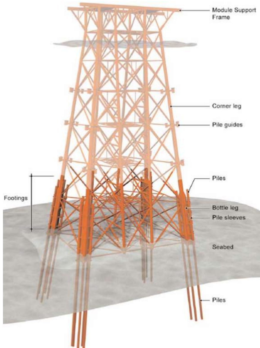
Figura 16 Struttura a torre con pali raggruppati
