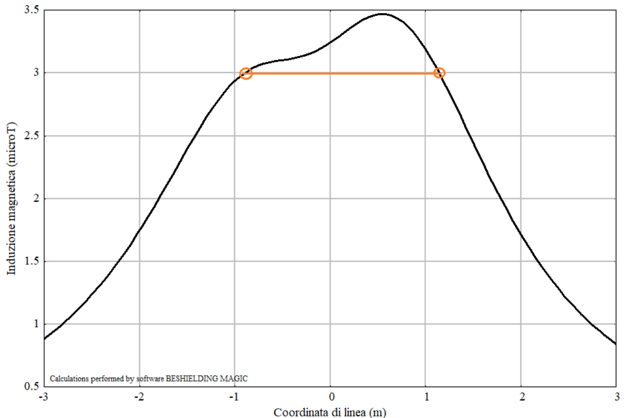
Figura 3. Valori dell'induzione magnetica B sul livello stradale (colore arancione: fascia di rispetto al suolo)
