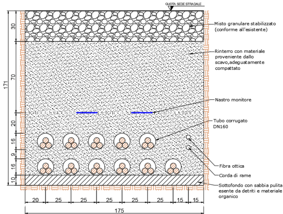
Figura 1. Sezione cavidotto MT a 30 kV composto da quattro linee di ingresso e cinque linee in uscita dalla cabina di raccolta
