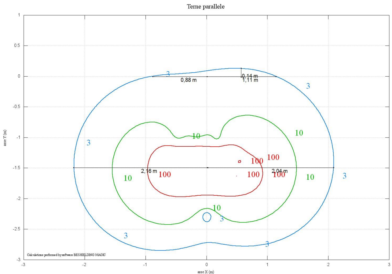
Figura 2. Curve di iso-campo dell'induzione magnetica B
