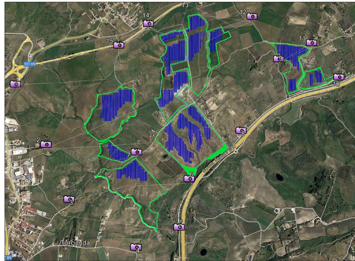
Punto di vista 12: Stato di progetto
