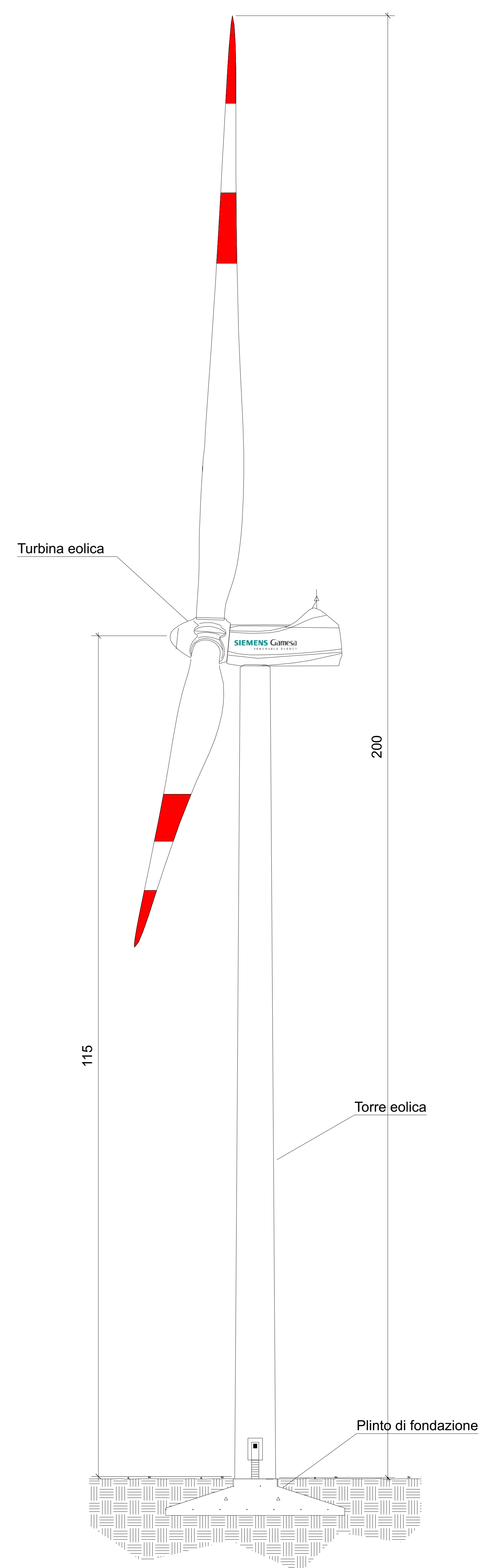
2 Prospetto laterale Scale: 1:300
