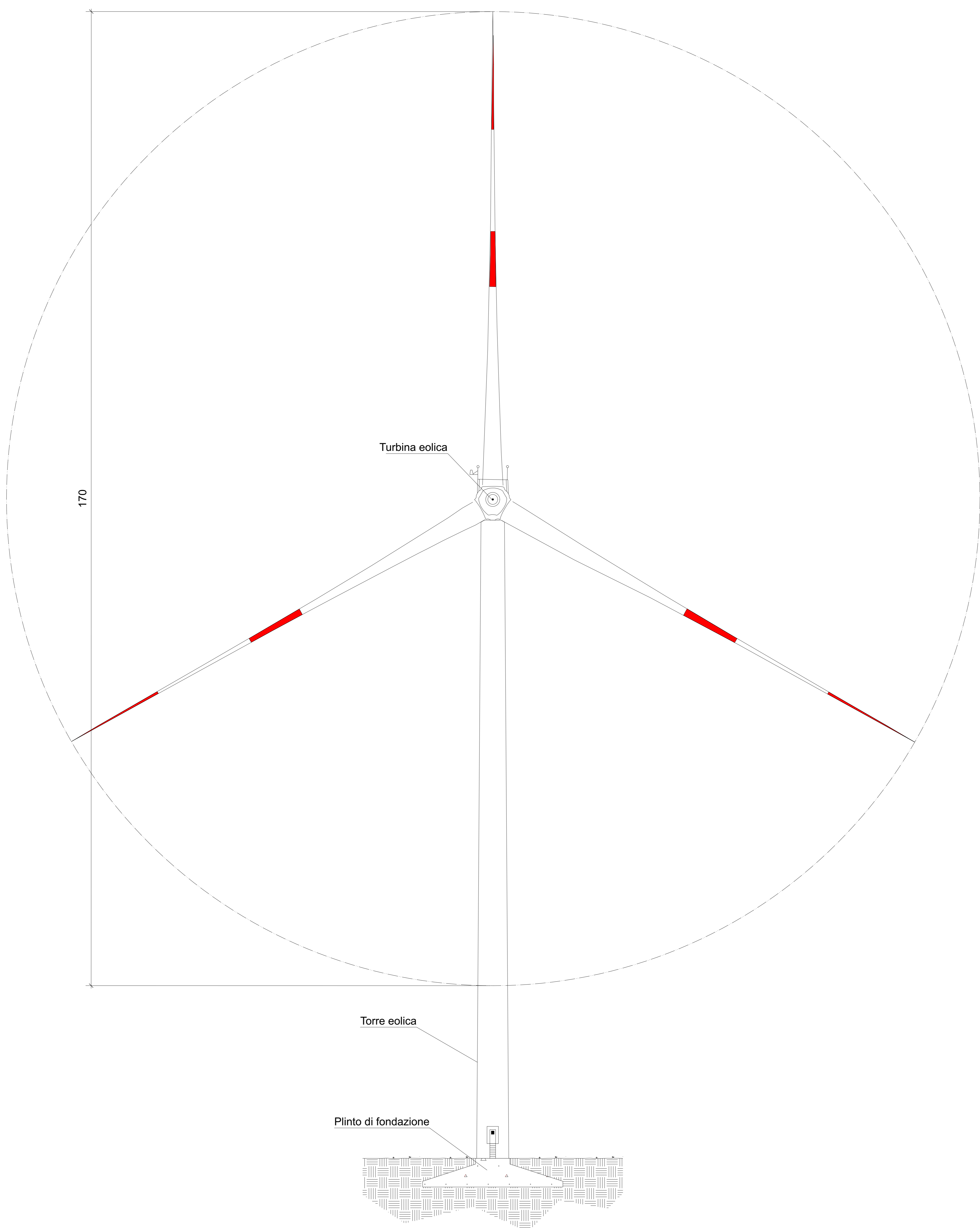
1 Prospetto frontale Scale: 1:300
