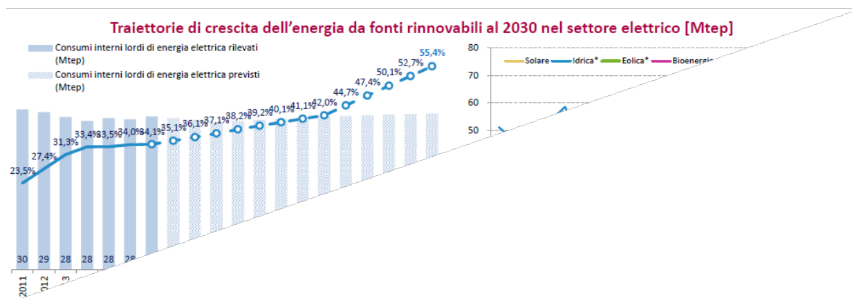
Traiettorie di crescita dell'energia da fonti rinnovabili al 2030 nel settore elettrico (Mtep) (*Fonte GSE)
