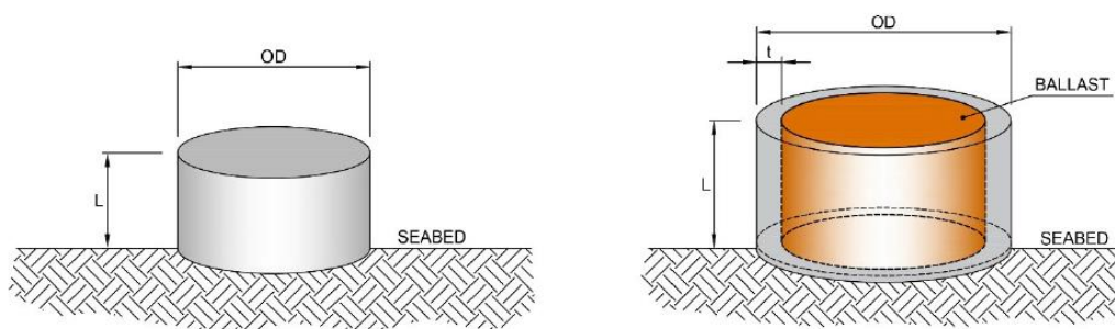
Figura 3.1: Schema Semplificato di Ancore a Gravità Piene (Sinistra) o Cave con Zavorra (Destra)
