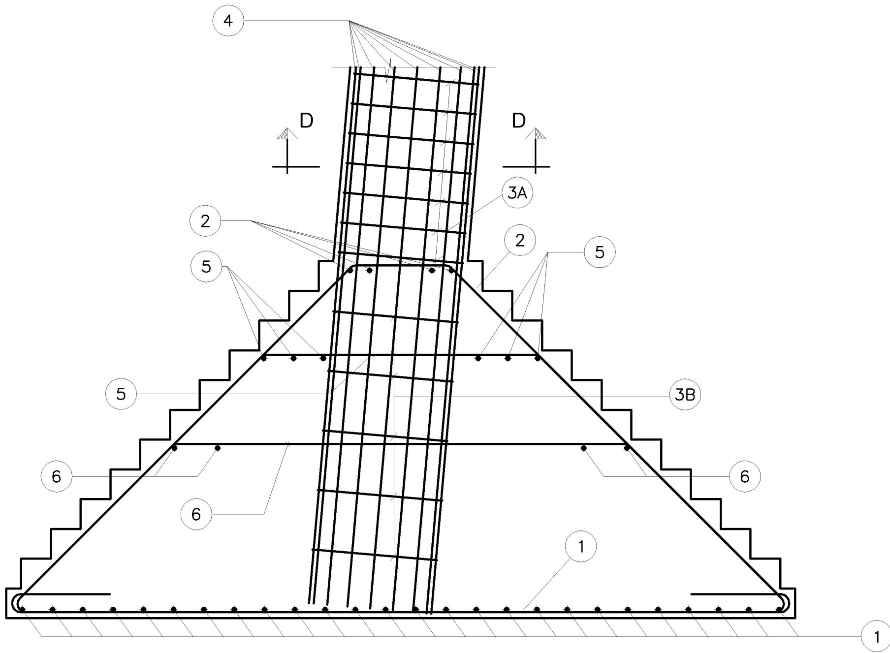
SEZIONE C-C 1:25
