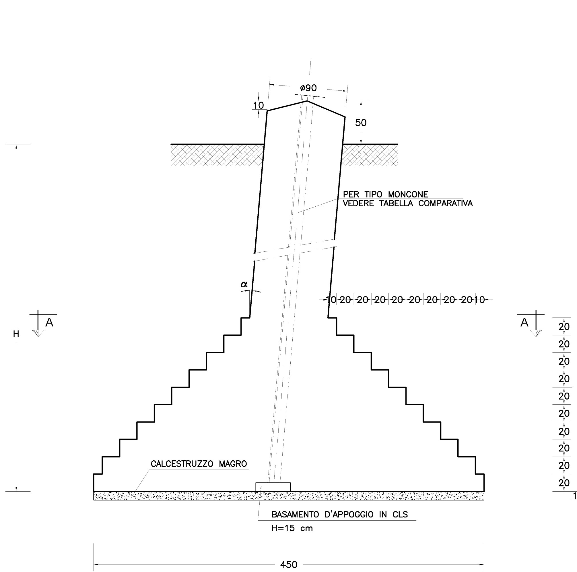
SEZIONE B-B 1:25
