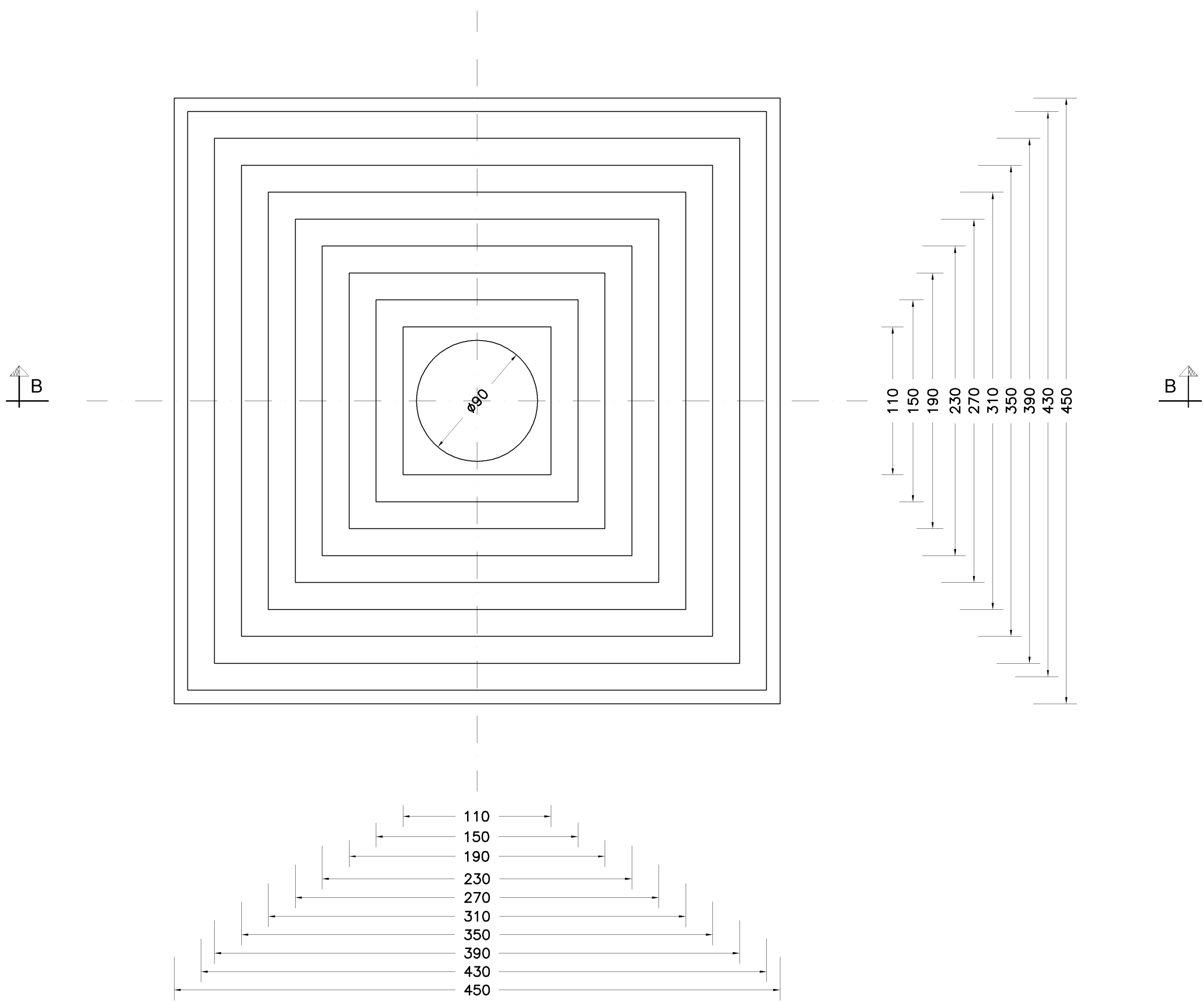
SEZ. A-A PLINTO DI FONDAZIONE 1:25
