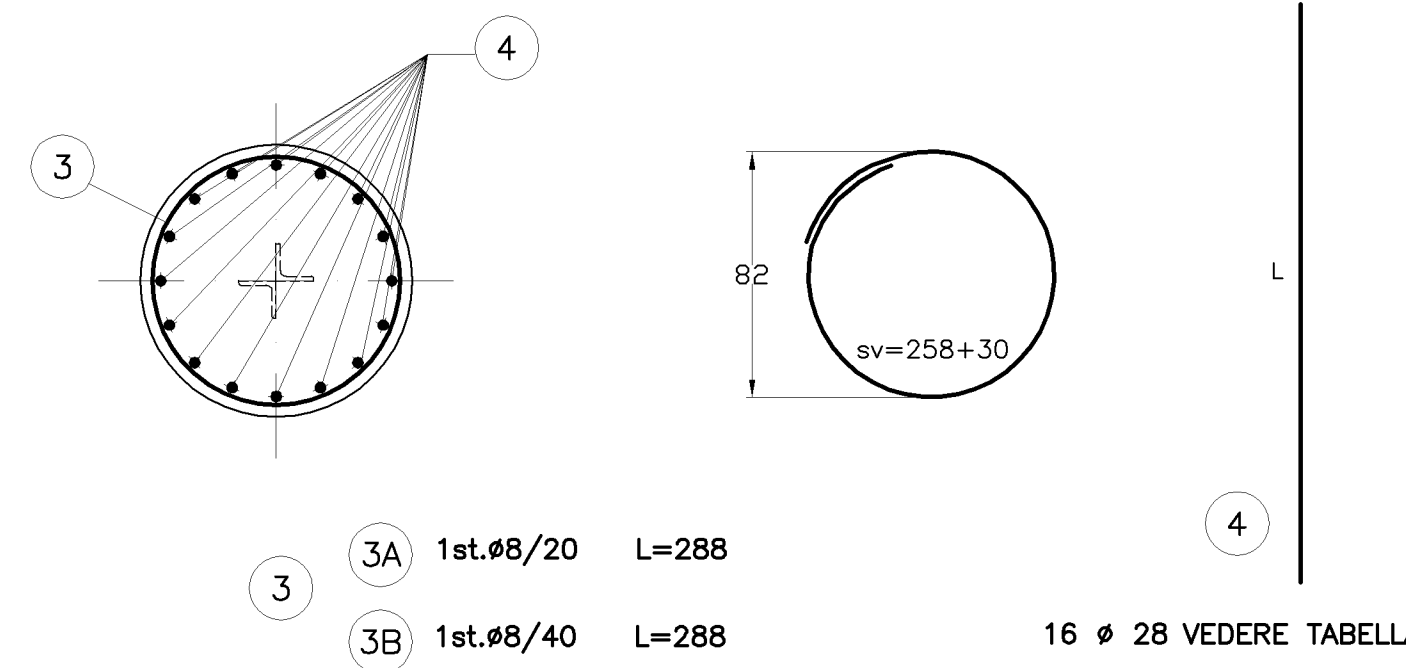
SEZIONE D-D 1:25
