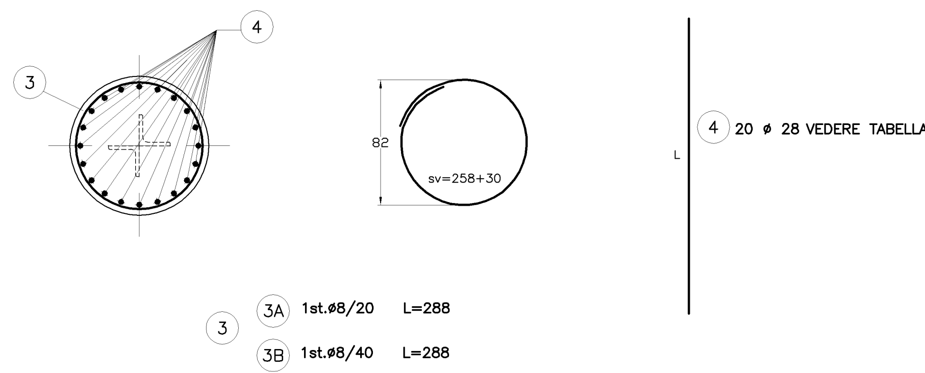
SEZIONE D-D 1:25
