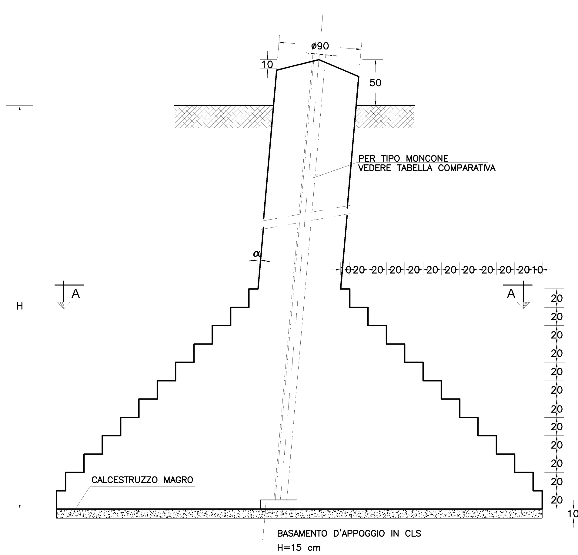
SEZIONE B-B 1:25
