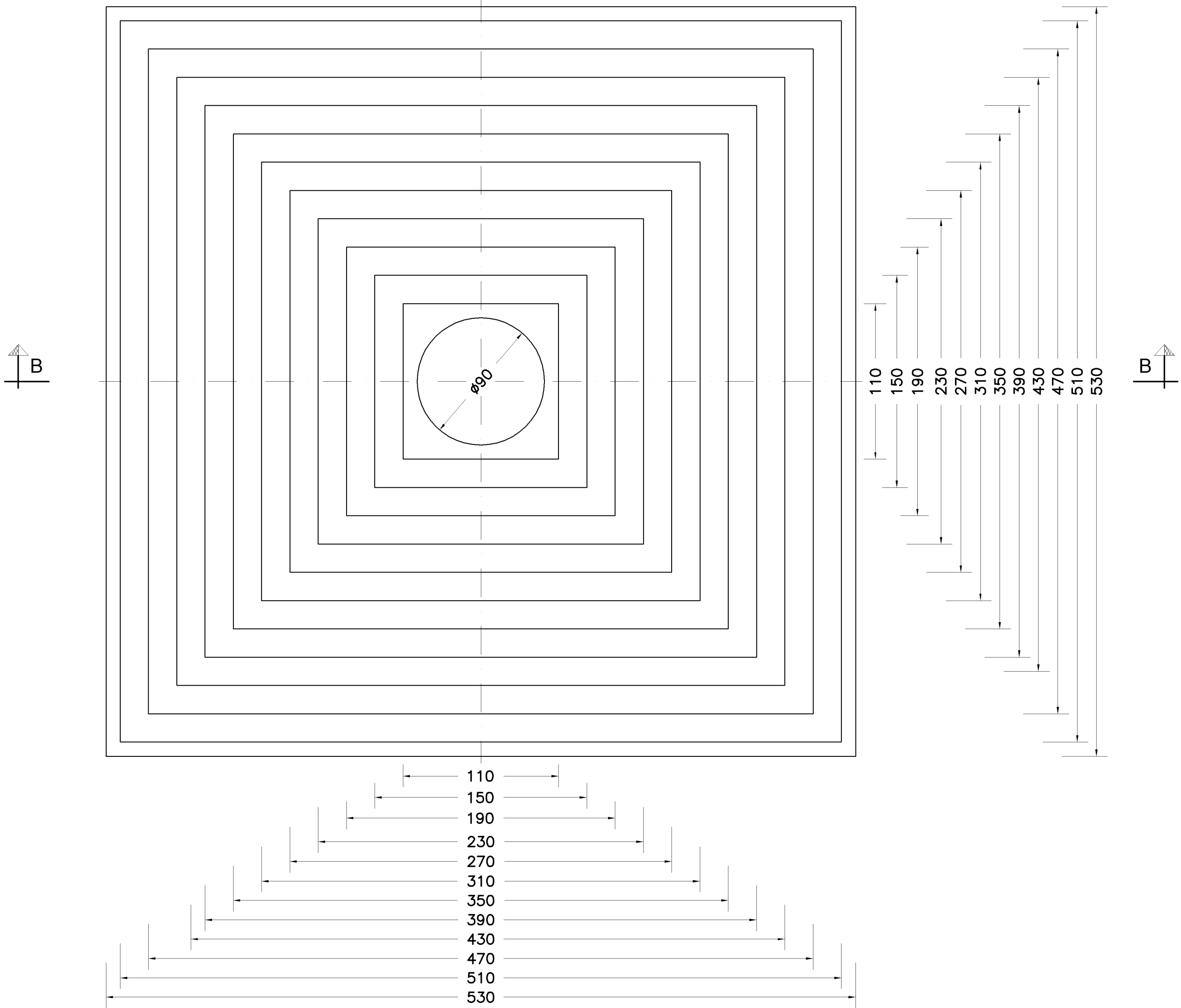
SEZ. A-A PLINTO DI FONDAZIONE 1:25
