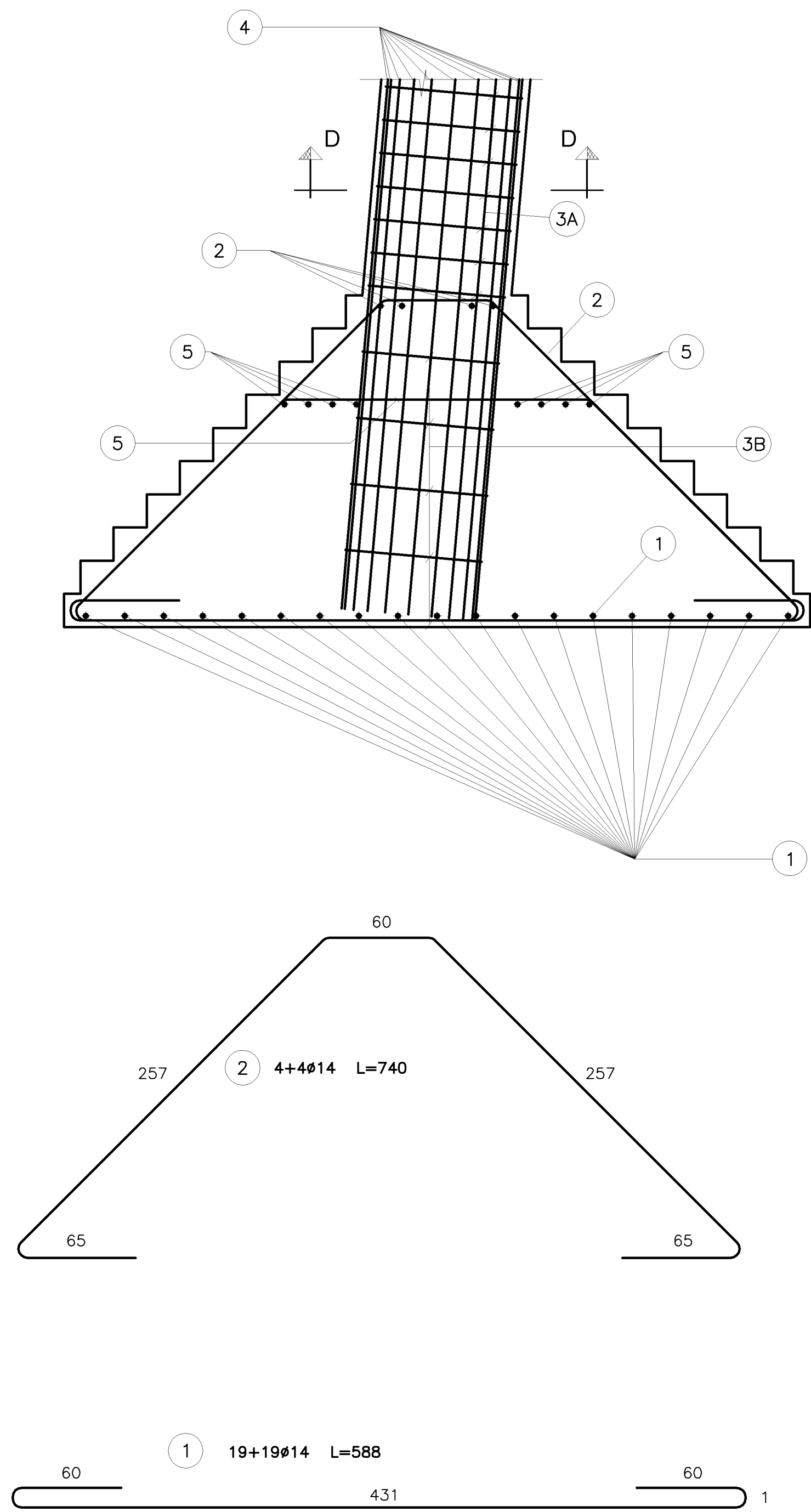
SEZIONE C-C 1:25
