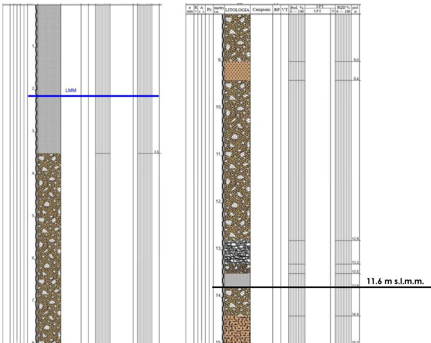
Figura 2-6. Stratigrafia del sondaggio C1.
