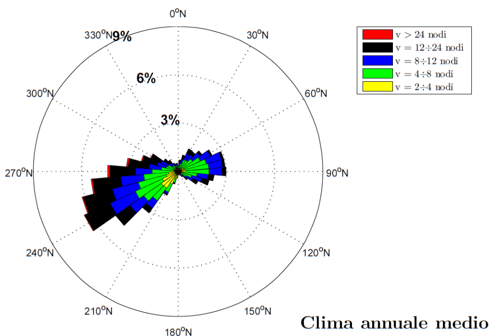
Figura 1-3 - Rappresentazione polare della distribuzione direzionale annuale degli eventi anemometrici nel Golfo di Olbia ottenuta sulla base delle misure effettuate presso l'aeroporto di Olbia.
