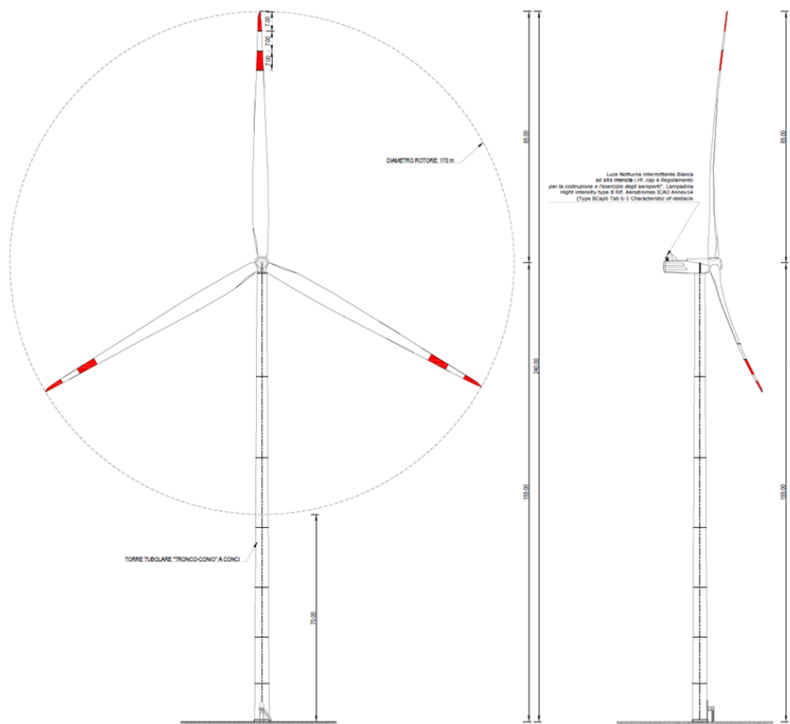
Figura 3 – Vista prospettica e laterale dell’aerogeneratore SIEMENS GAMESA SG 6.6- 170 da max 6,6 MW
