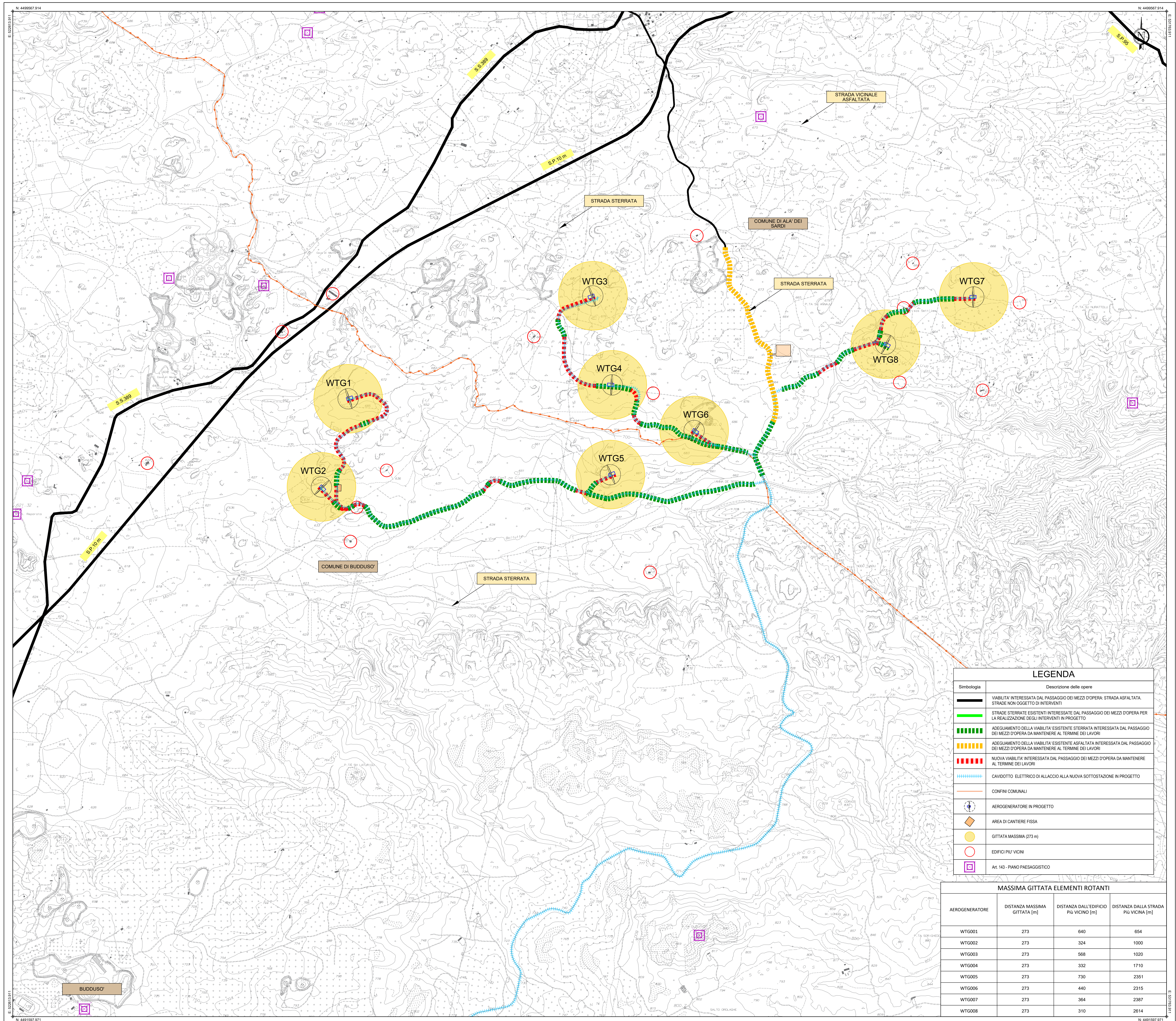
TAVOLA GRAFICA DELLA GITTATA MASSIMA - ELEMENTI ROTANTI Base carta: Carta Tecnica Regionale 1:10.000
