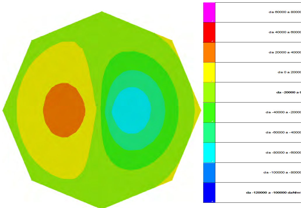
Figura 5 - Rappresentazione in pianta delle massime compressioni sul terreno in famiglia SLU.
