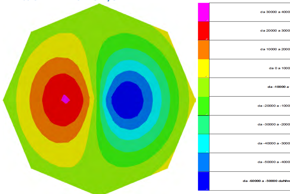
Figura 7 - Rappresentazione in pianta delle massime compressioni sul terreno in famiglie SLE/SLD.
