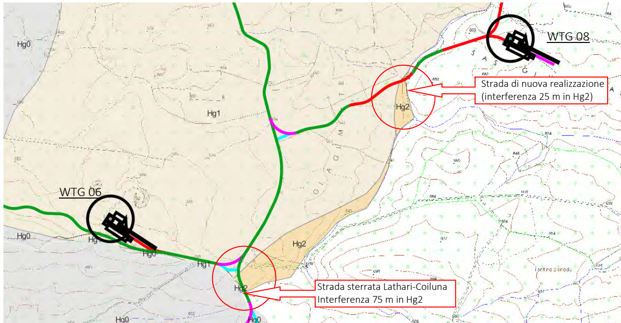
Figura 1 – Particolare della tavola Allegato 1 in cui si evidenzia, cerchiati in rosso, i due punti dell'attraversamento del cavidotto in aree Hg2
