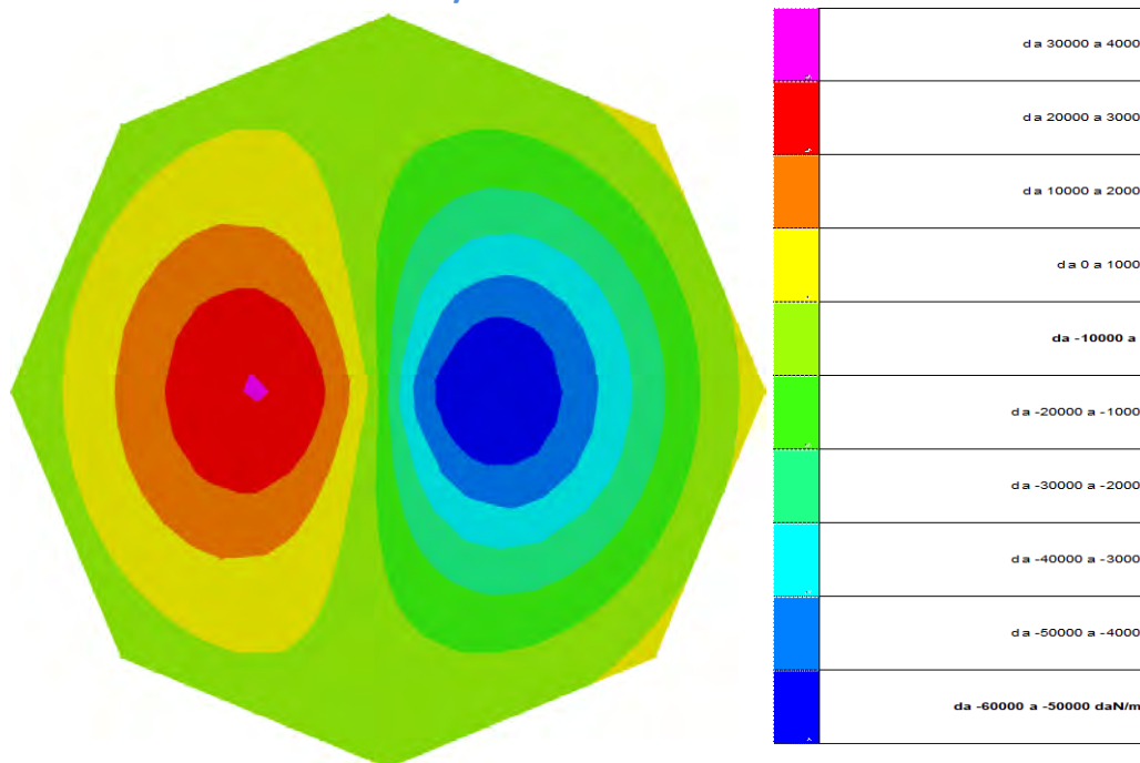
Figura 6 - Rappresentazione in pianta delle massime compressioni sul terreno in famiglie SLVf/SLUEcc.
