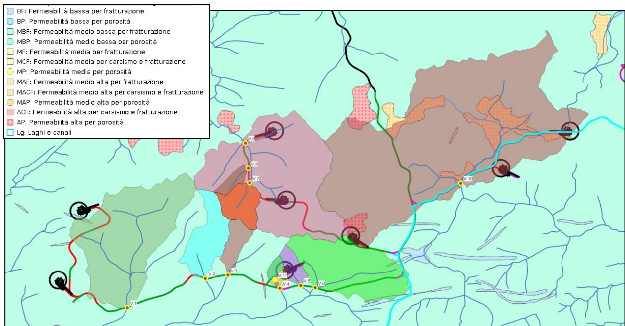
Figura 11 – Carta della permeabilità dei substrati della Sardegna per il territorio in analisi
