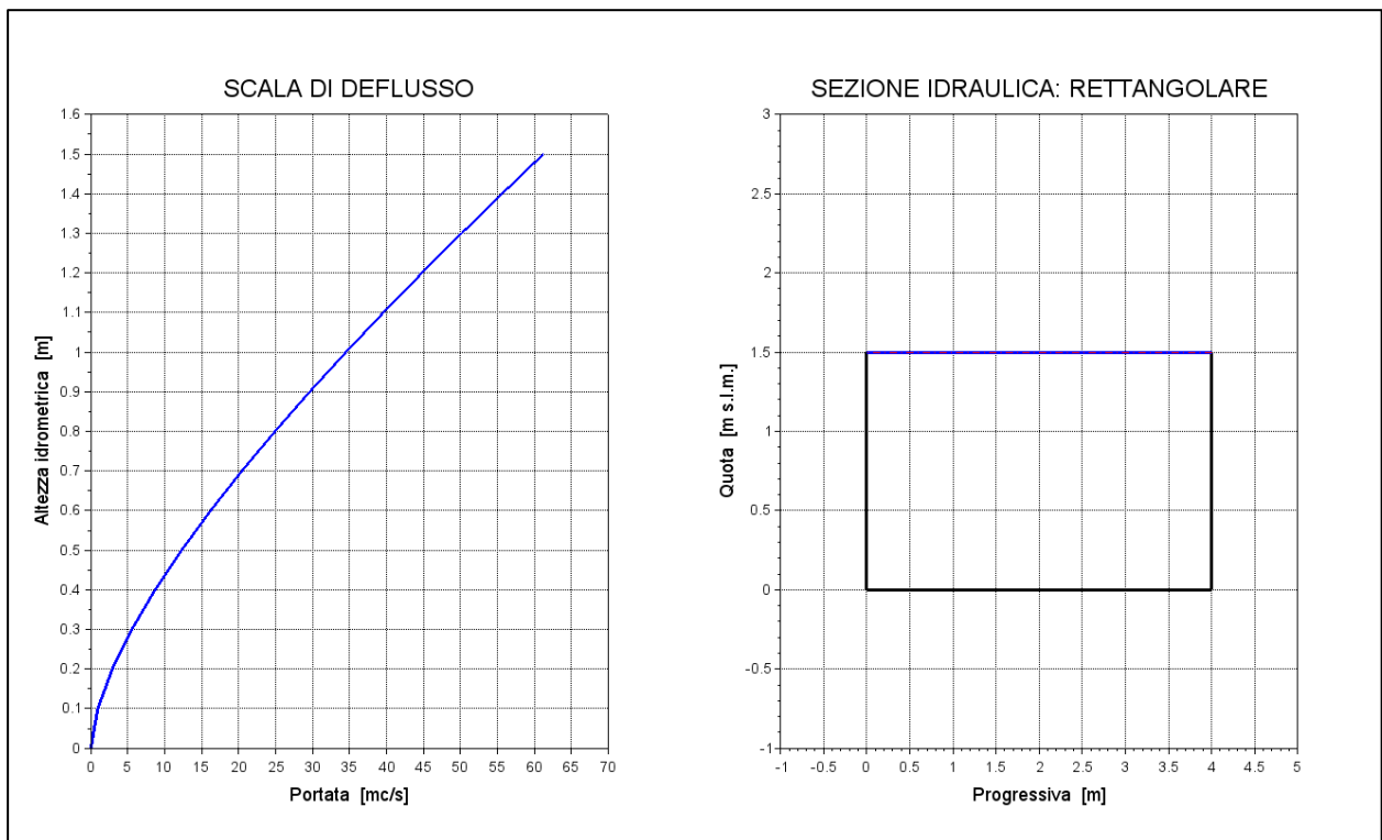
Figura 14 – Scale di deflusso di moto uniforme per gli elementi scatolari di dimensioni 2,0 x 1,5 m e 4,0 x 1,5 m.
