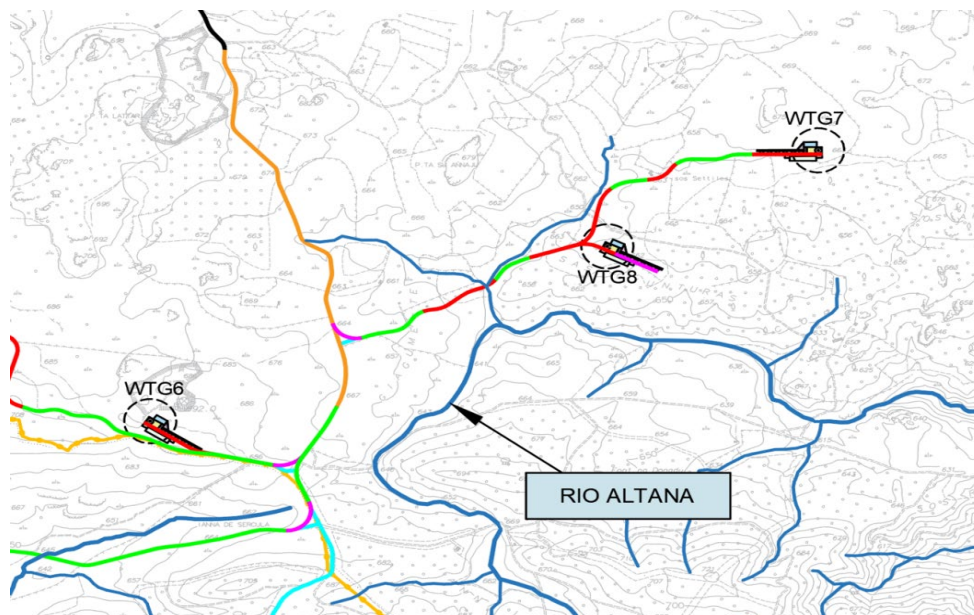
Figura 8 – Viabilità interna parco eolico “Buddusò Sud I” per l’accesso agli aerogeneratori WTG 6-7-8 (in arancione strada solo da allargare, in verde le piste esistenti oggetto di solo adeguamento e in rosso i tratti di pista di nuova viabilità; in magenta tratti di pista di cantiere da rimuovere a fine lavori per ripristinare paesaggio presente)
