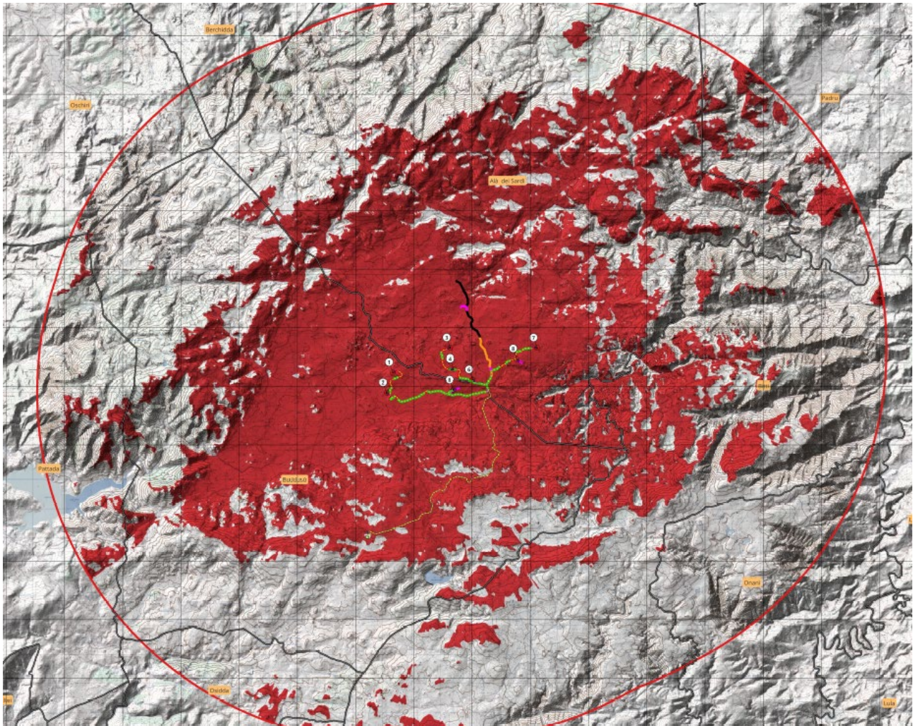
Figura 23 - Mappa di intervisibilità teorica del solo impianto eolico in progetto - (calcolata su base orografica)
