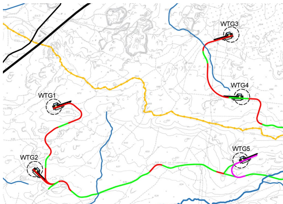
Figura 9 - Viabilità interna parco eolico “Buddusò Sud I” per l’accesso agli aerogeneratori WTG 1-2-3-4-5.
