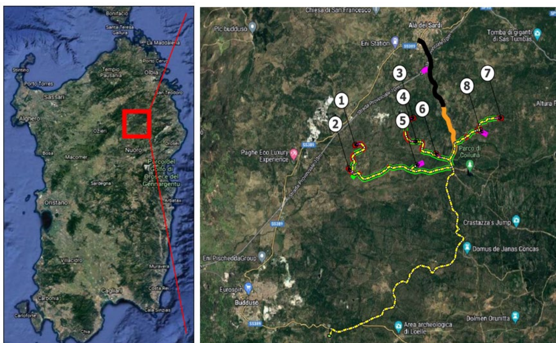
Figura 1 - Inquadramento del Parco eolico - fonte Google Earth
