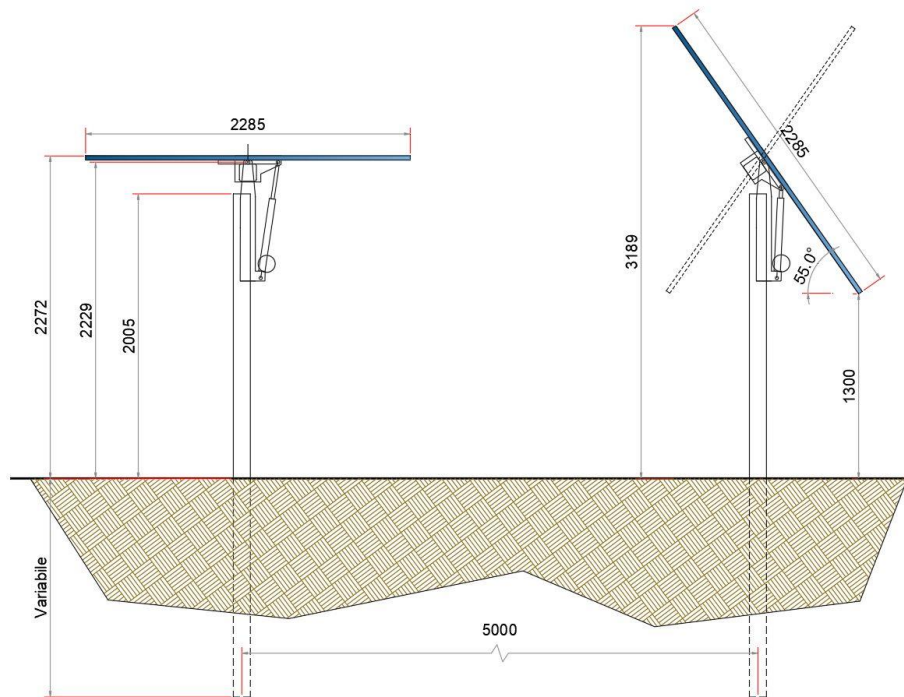
Fig. 3- Tracker - Inseguitore mono-assiale - intervalli di rotazione
