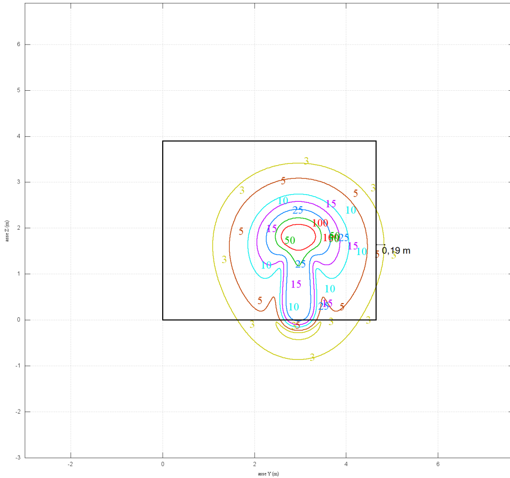
Cabina - calcolo su piano yz - quote X=9,24 m
