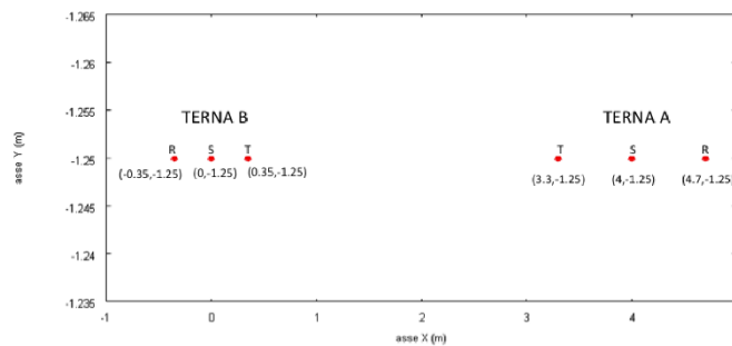
Figura 5: Geometria sorgenti
