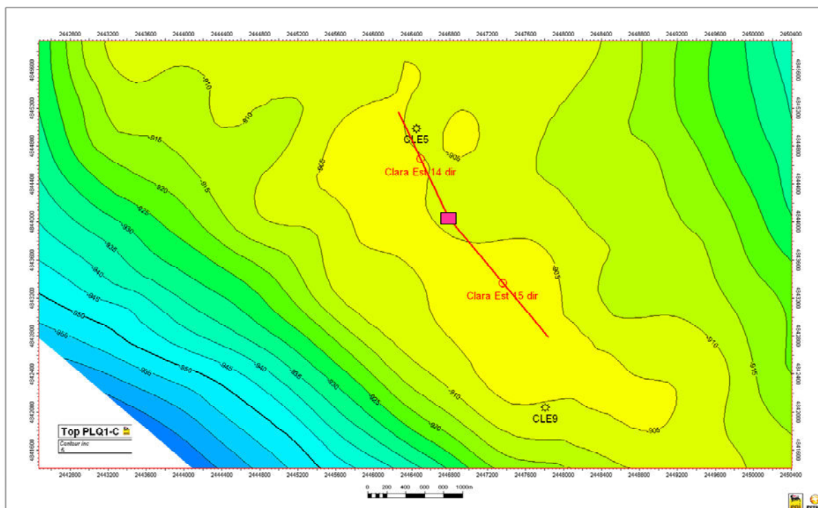
Figura 3 – Ubicazione dei pozzi di sviluppo di Clara Sud-Est.
