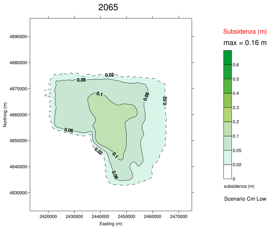
Figura 22 – Curve di iso-subsidenza per lo scenario Cm_Lower al 2065.
