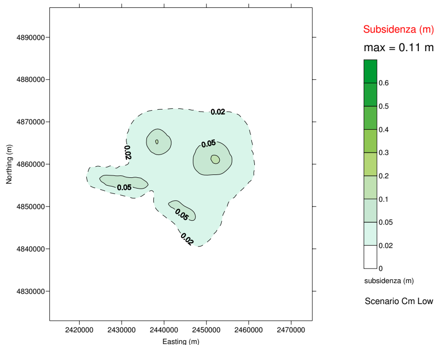
Figura 18 – Curve di iso-subsidenza per lo scenario Cm_Lower al 2013.
