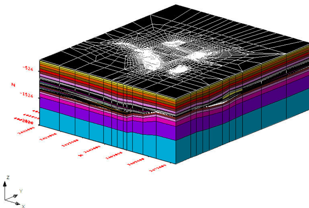
Figura 4 – Griglia di calcolo ad elementi finiti utilizzata nel modello geomeccanico Isamgeo. La scala verticale della rappresentazione è pari a 10 volte quella orizzontale.
