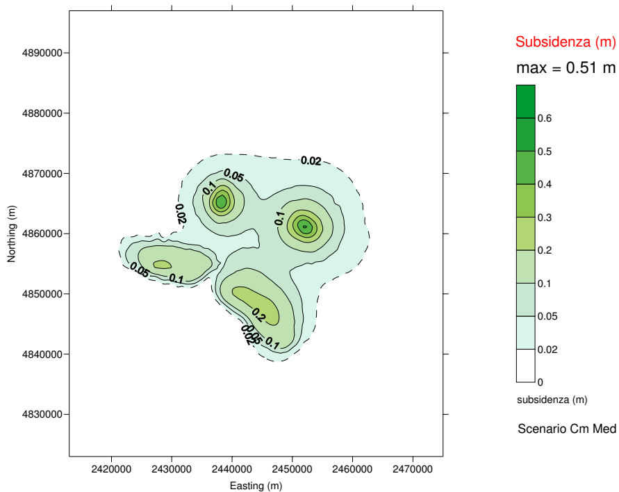
Figura 8 – Curve di iso-subsidenza per lo scenario Cm_Med al 2013.
