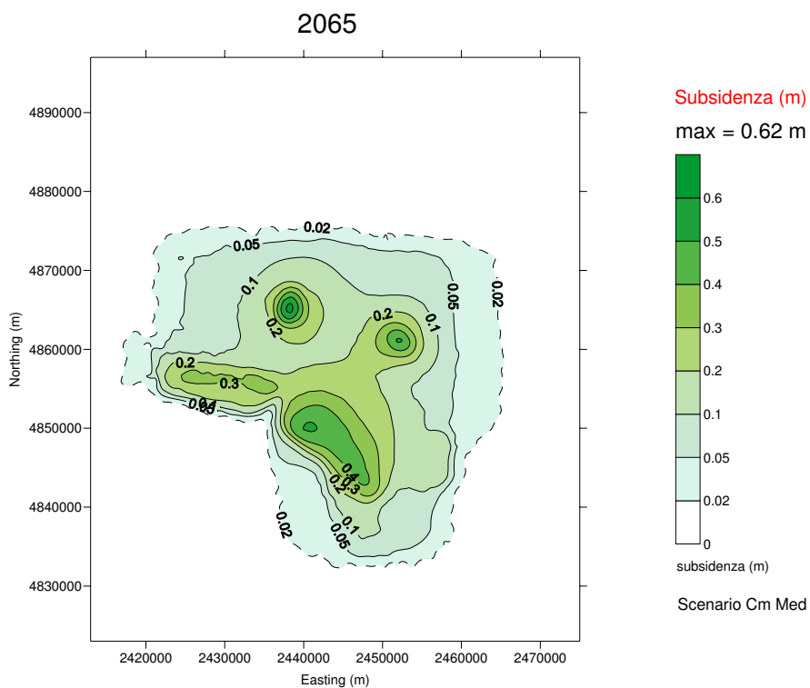
Figura 12 – Curve di iso-subsidenza per lo scenario Cm_Med al 2065.
