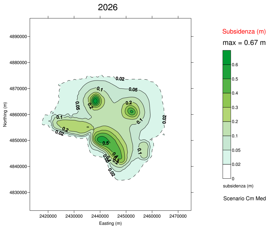
Figura 10 – Curve di iso-subsidenza per lo scenario Cm_Med al 2026.
