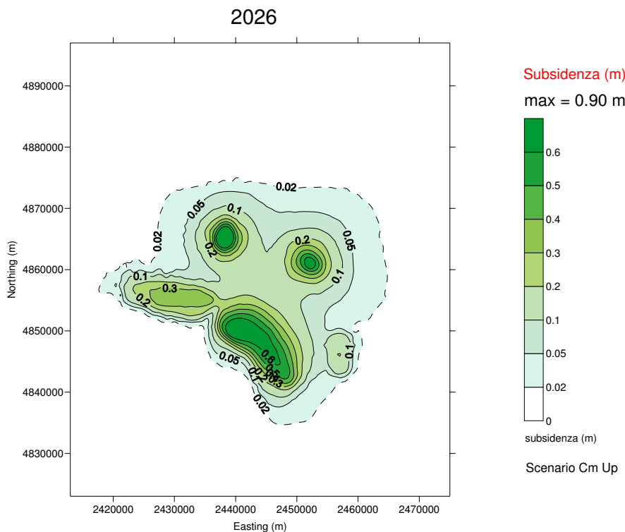
Figura 15 – Curve di iso-subsidenza per lo scenario Cm_Upper al 2026.
