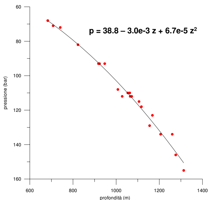
Figura 6 – Pressioni iniziali relative all'insieme dei campi del Clara Complex, Calipso ed Elettra.
