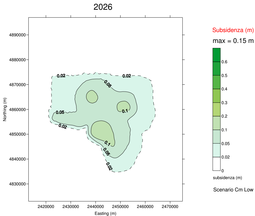
Figura 20 – Curve di iso-subsidenza per lo scenario Cm_Lower al 2026.
