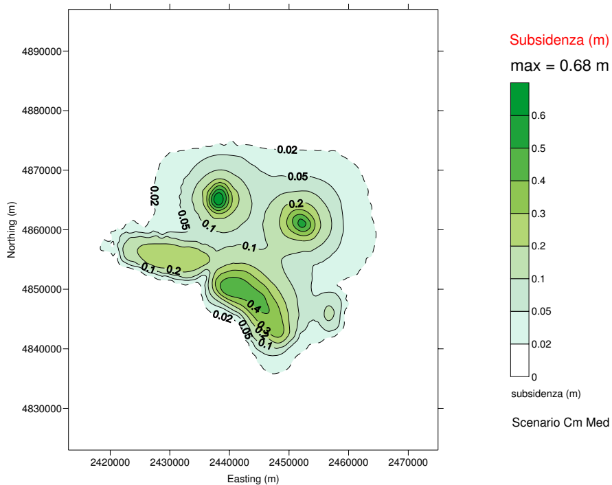
Figura 9 – Curve di iso-subsidenza per lo scenario Cm_Med al 2021.
