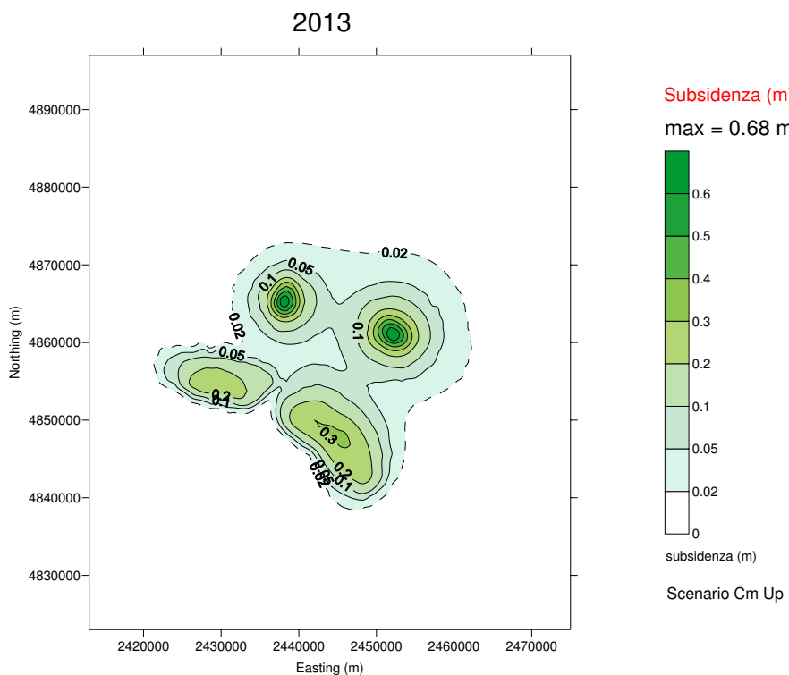
Figura 13 – Curve di iso-subsidenza per lo scenario Cm_Upper al 2013.
