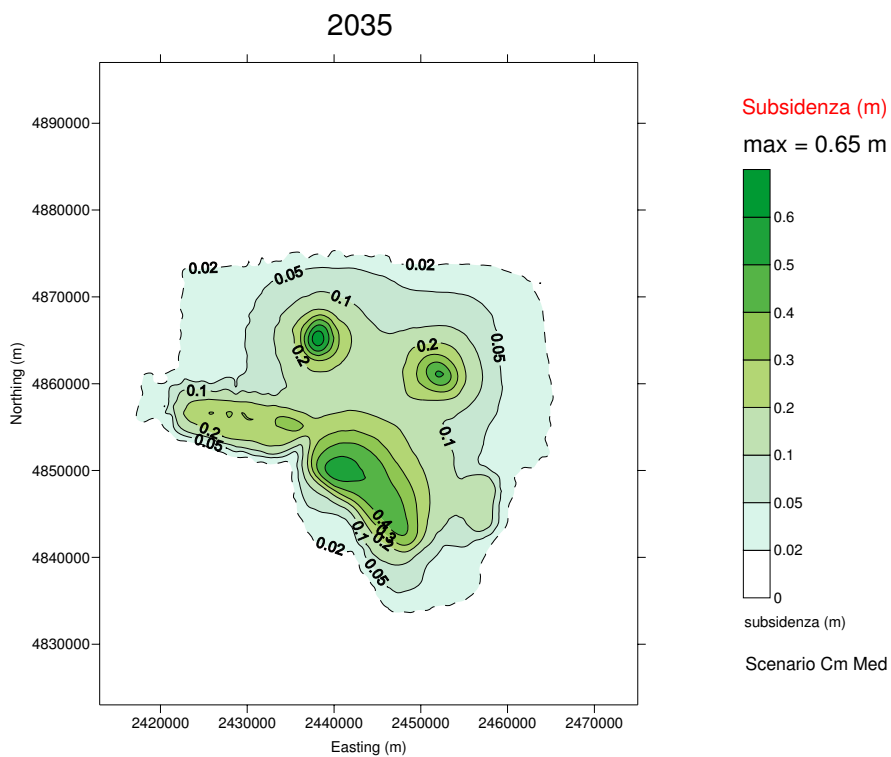
Figura 11 – Curve di iso-subsidenza per lo scenario Cm_Med al 2035.
