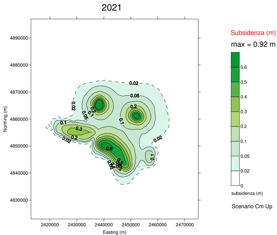
Figura 14 – Curve di iso-subsidenza per lo scenario Cm_Upper al 2021.
