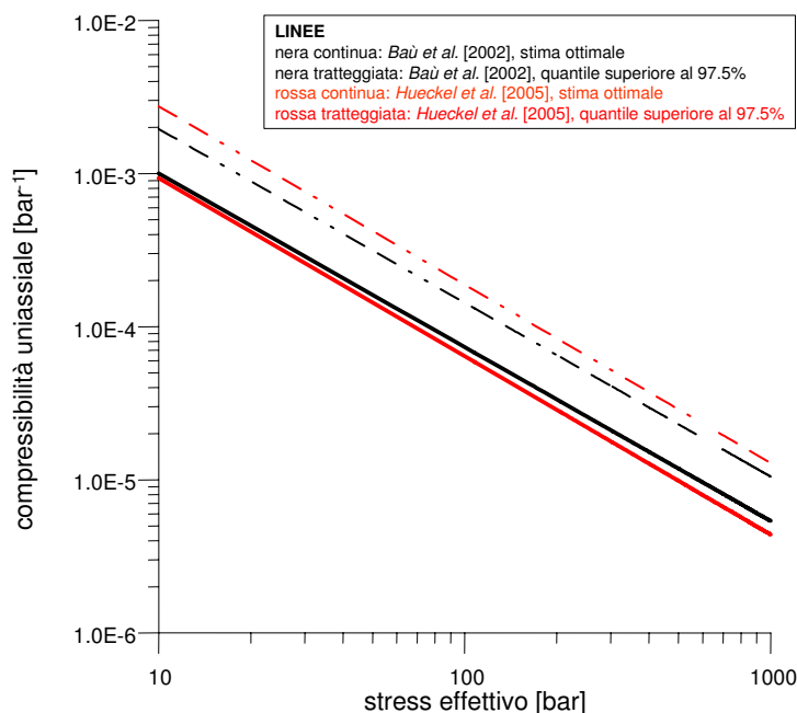
Figura 5 – Correlazione tra la compressibilità uniassiale c_m e lo stress efficace in situ, derivata da misure su marker nei campi a gas del bacino nord adriatico (da [3]).
