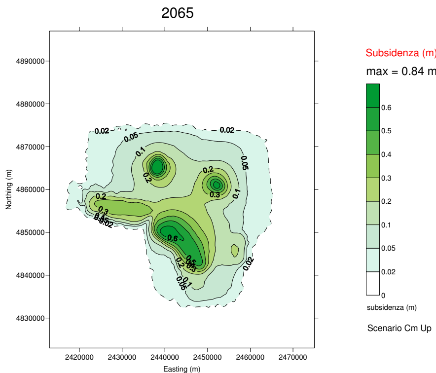
Figura 17 – Curve di iso-subsidenza per lo scenario Cm_Upper al 2065.
