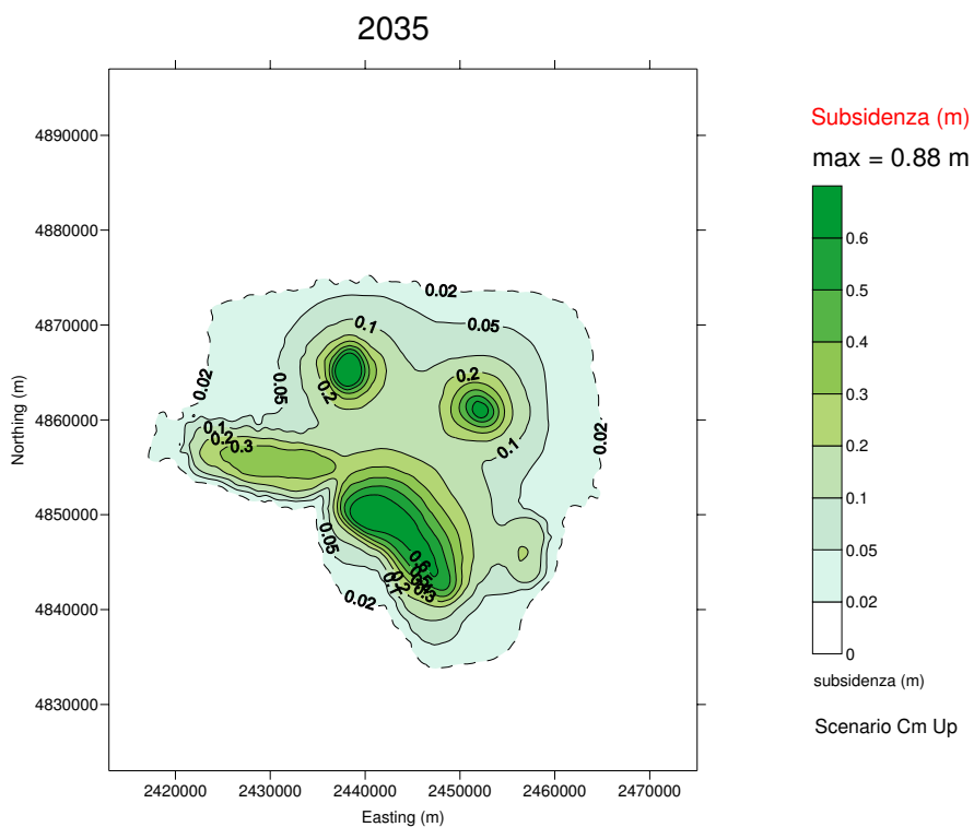
Figura 16 – Curve di iso-subsidenza per lo scenario Cm_Upper al 2035.
