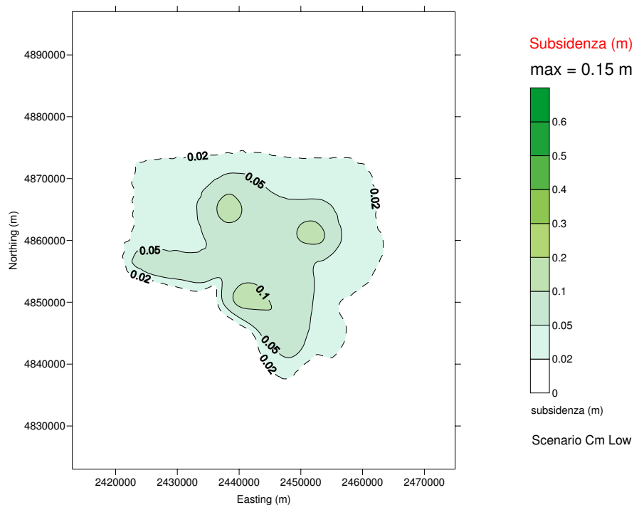
Figura 19 – Curve di iso-subsidenza per lo scenario Cm_Lower al 2021.
