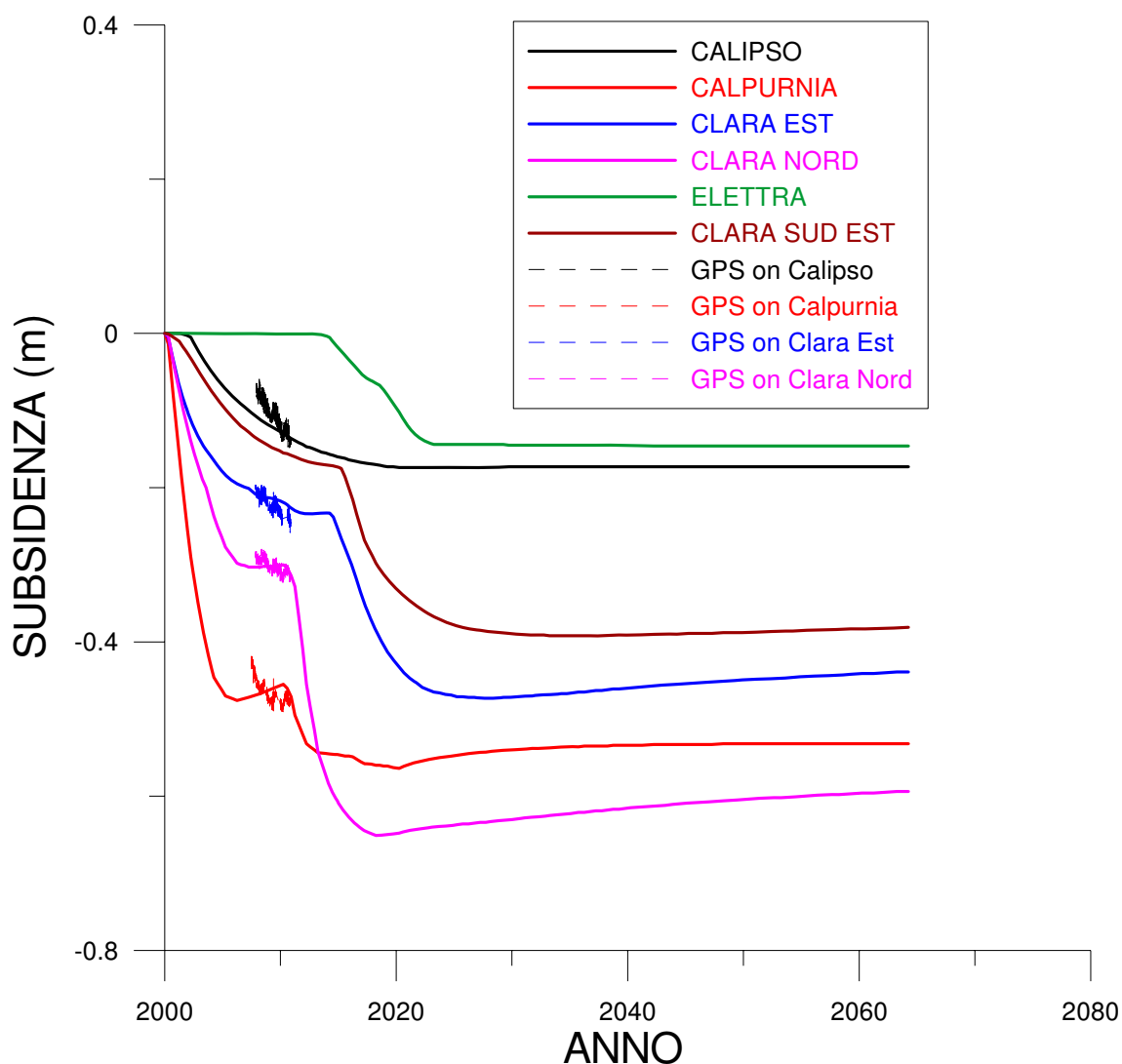
Figura 7 – Andamento temporale della subsidenza prevista nello scenario Cm_Med nei 6 punti di controllo corrispondenti alle piattaforme di produzione. Per Clara Nord, Clara Est, Calpurnia e Calipso le previsioni di subsidenza sono confrontate con le misure di subsidenza ottenute tramite GPS in continuo.
