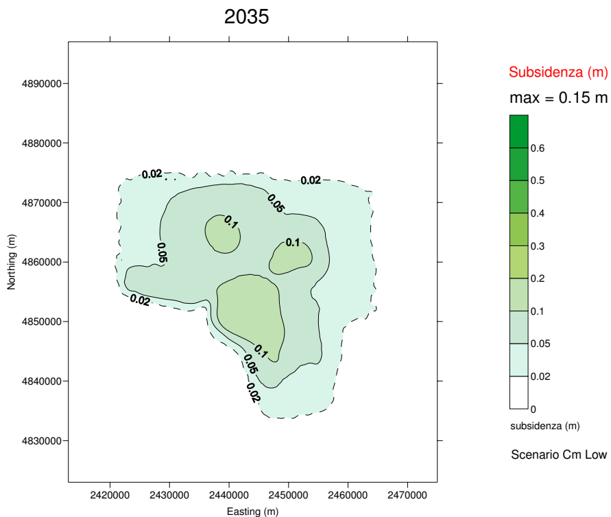
Figura 21 – Curve di iso-subsidenza per lo scenario Cm_Lower al 2035.
