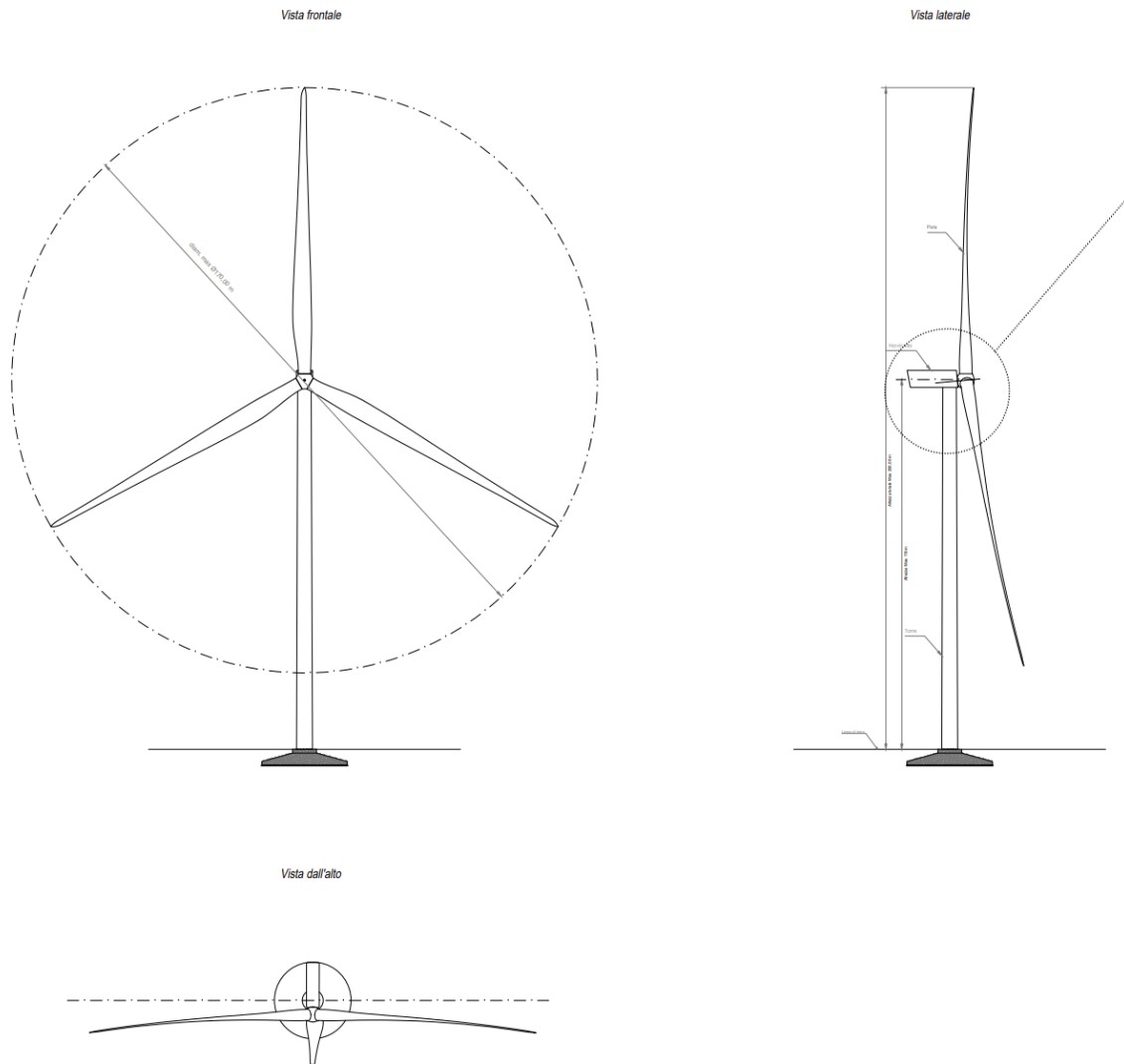
Figura 1 – Aerogeneratore tipo
