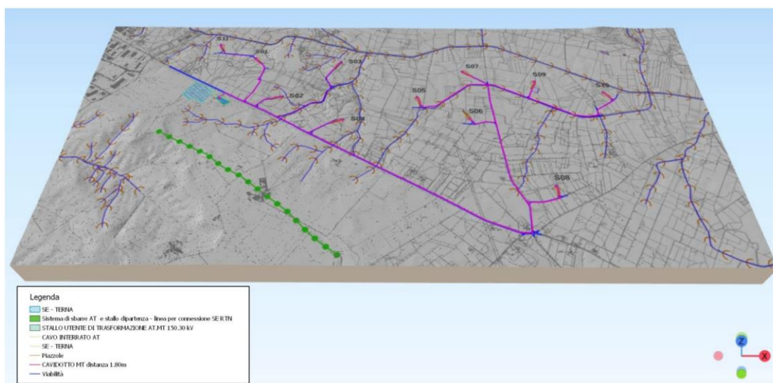
Figura 7 - Strutture geomorfologiche presenti su base DTM
