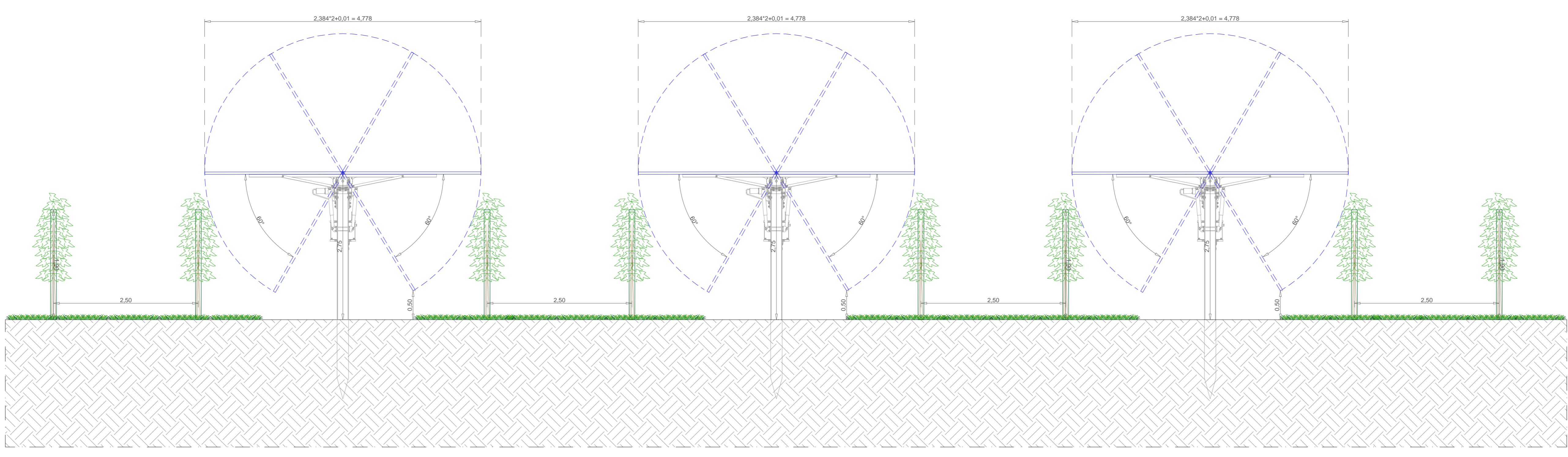
SEZIONE TIPOLOGICA IMPIANTO AGROVOLTAICO - SCALA DI RIPRODUZIONE 1:40
