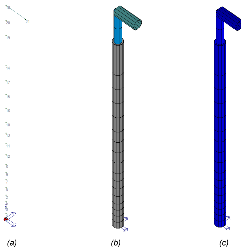
Figura 2 - Schema del modello strutturale unipylon (a) con indicazione dei nodi, schema con individuazione delle sezioni (b) e dei materiali (c)
