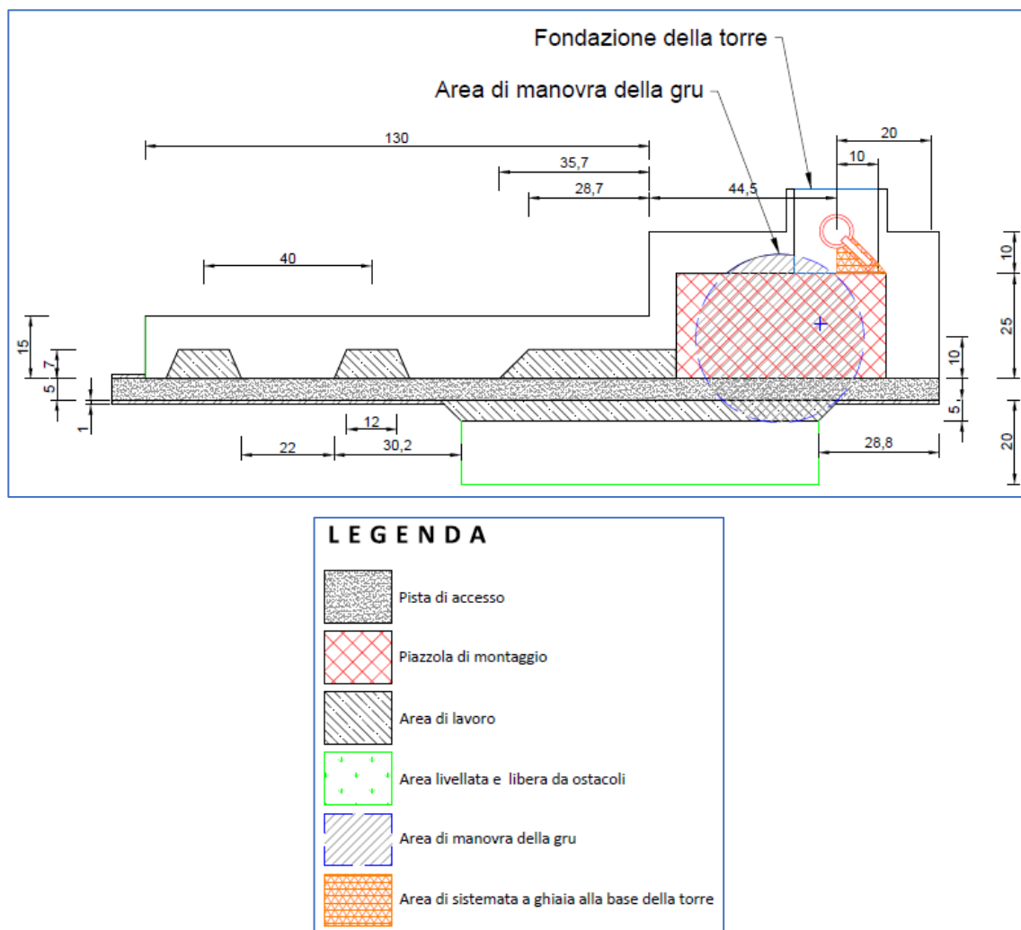
Figura 15 – tipologico della piazzola di montaggio
