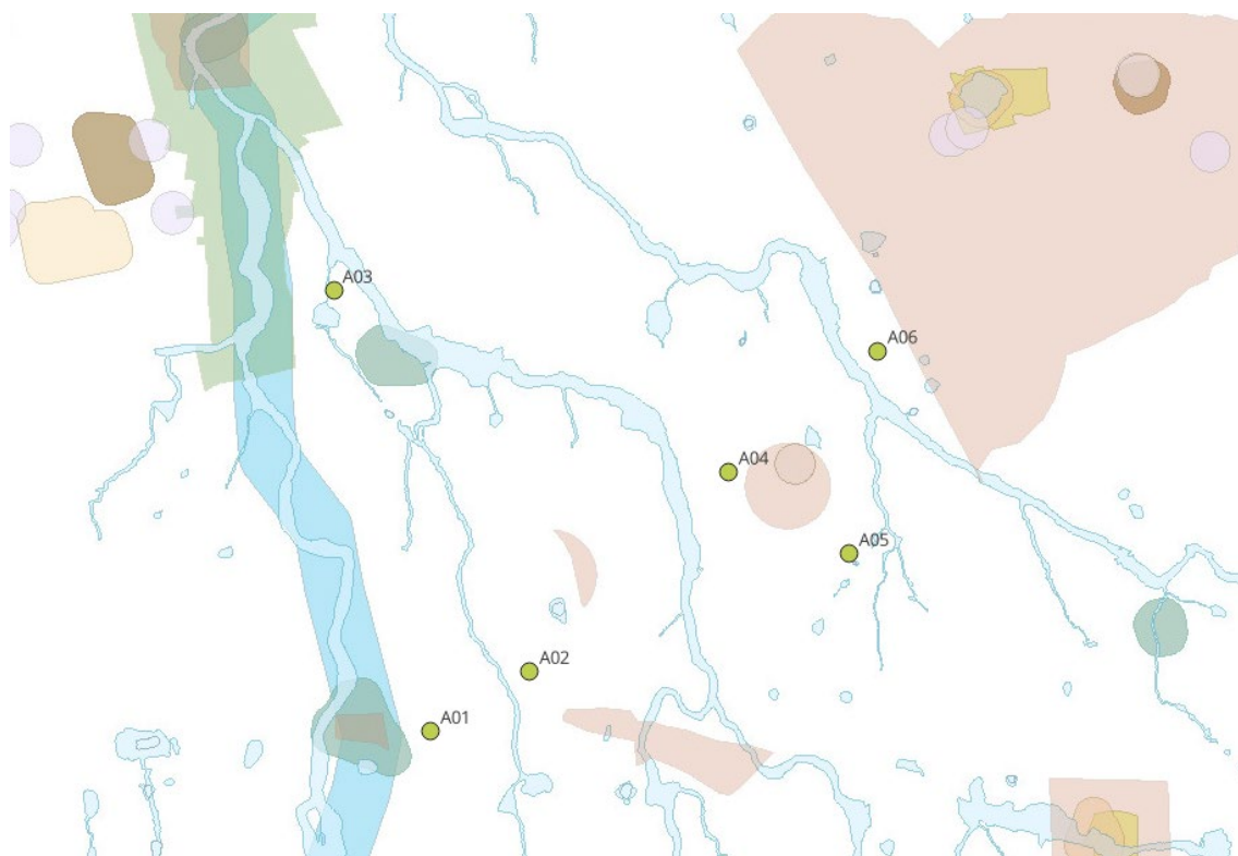
Figura 4 - Ipotesi Layout a 6 aerogeneratori con collocazione differente - analisi aree non idonee FER
